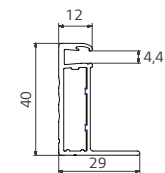
Frame Dwarsdoorsnede
