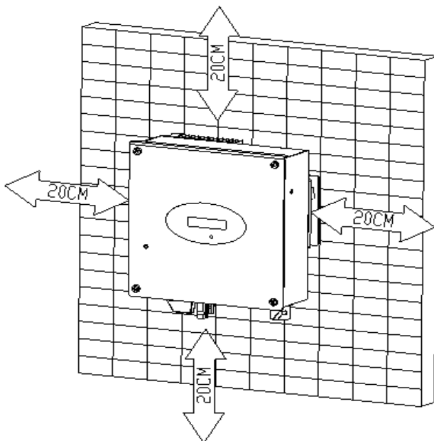
Afmetingen ten opzichte van de omgeving voor één omvormer
