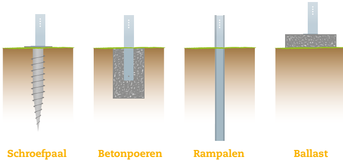
Schroefpaal
