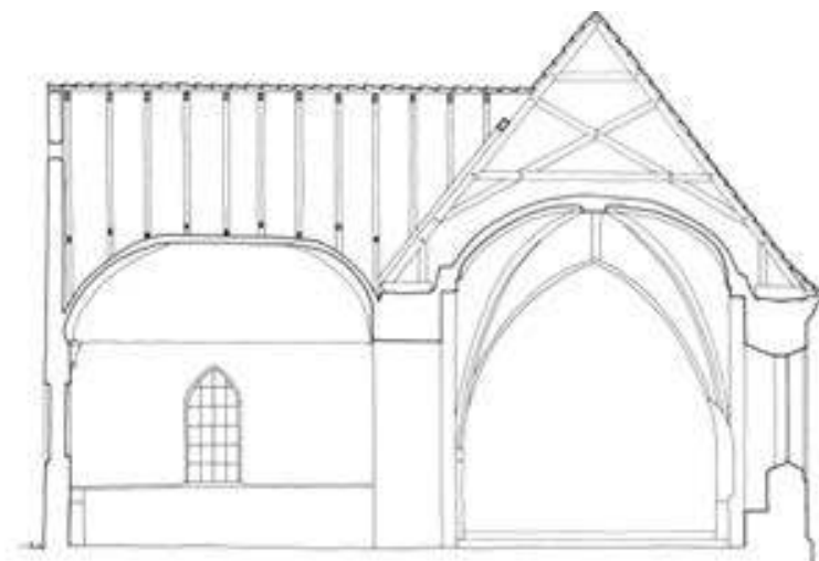
"Ombygget" kirke med murede hvælv (bort skarrede bjælker)
