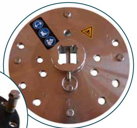
Universal hovedhjul med 5 stk styrebolte. Set fra top og bund.
