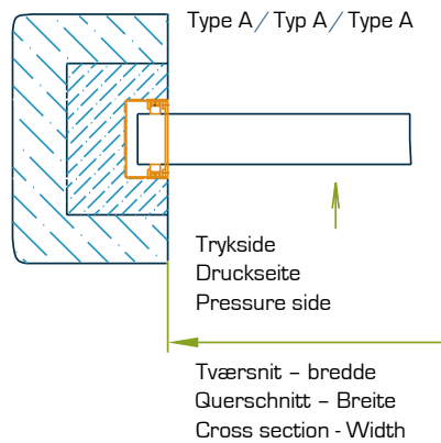
Typen af u-profiler Typen von Wandanschlussprofilen Types of lateral guide
