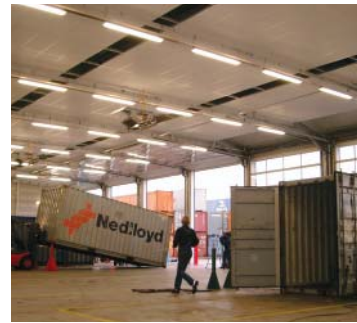
Werkhalle mit nichtbrennbarer Akustikdecke und Hinterlüftung zur Vermeidung einer Taupunktverschiebung (Kondenswasser).
