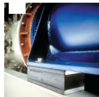
SCHWINGMETALL® Elemente
