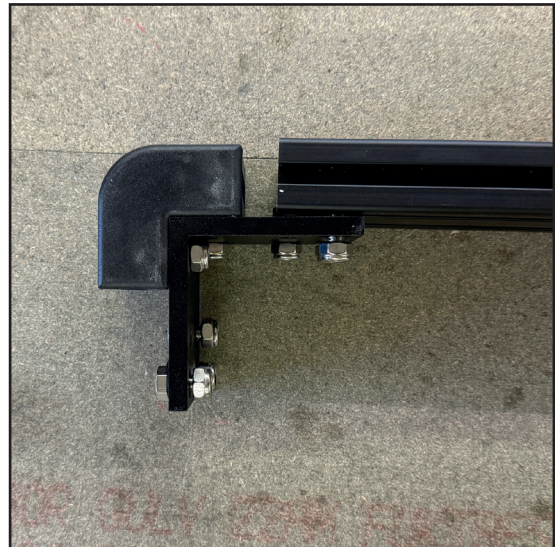
Sett hjørne fast på den korteste rammeprofilen
