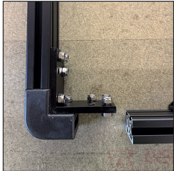
Sett til slutt på kortsidene med hjørner.
