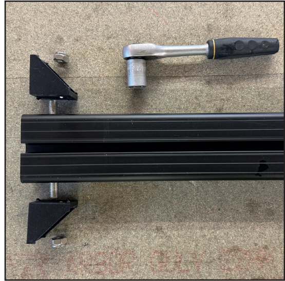
Monter festebrakettene med mutter og skrue, strammes med 13mm skralle.
