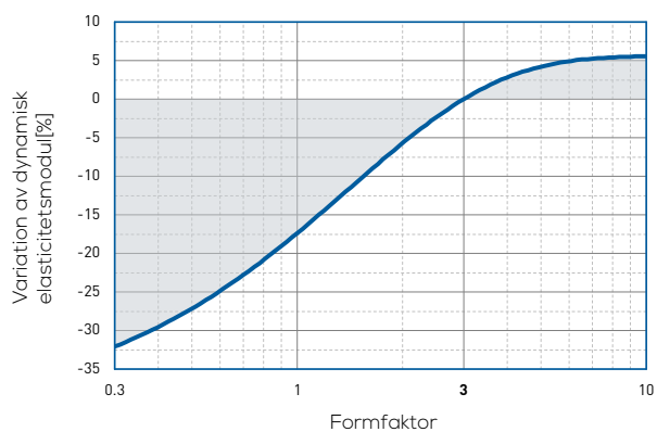
Dynamisk elasticitetsmodul at 10 Hz
