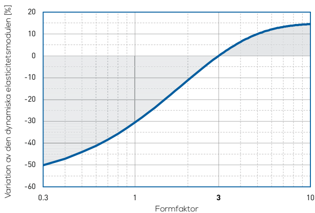
Dynamisk elasticitetsmodul vid 10 Hz
