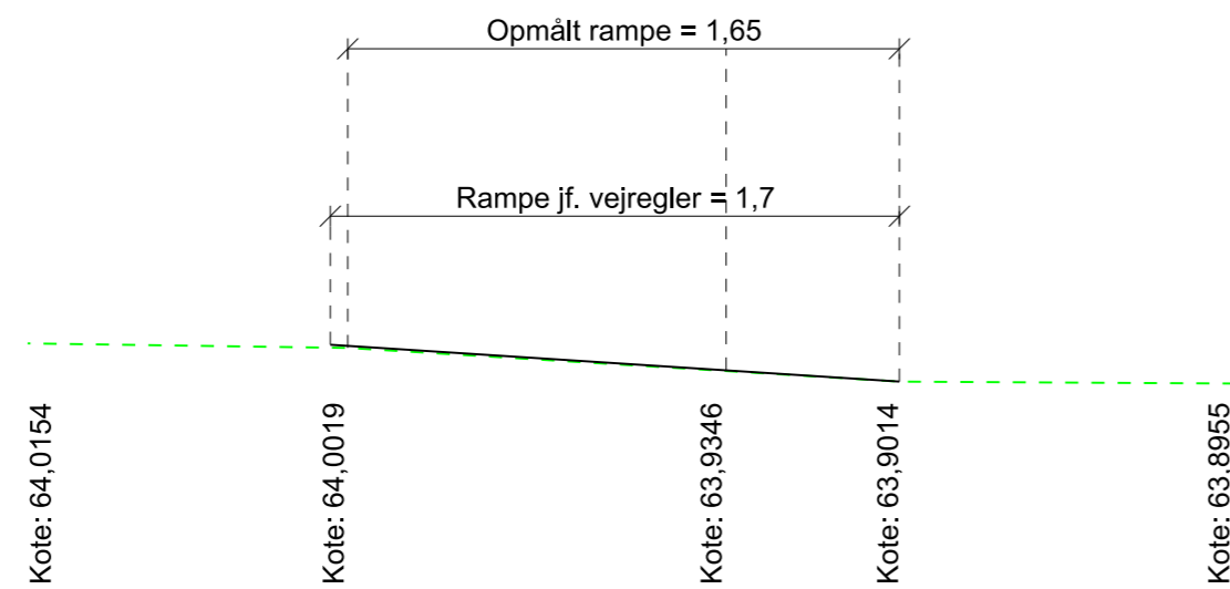
Snit F-F, 1:25 Snit igennem hævet flade nr. 02 Nordøstlig vejgren
