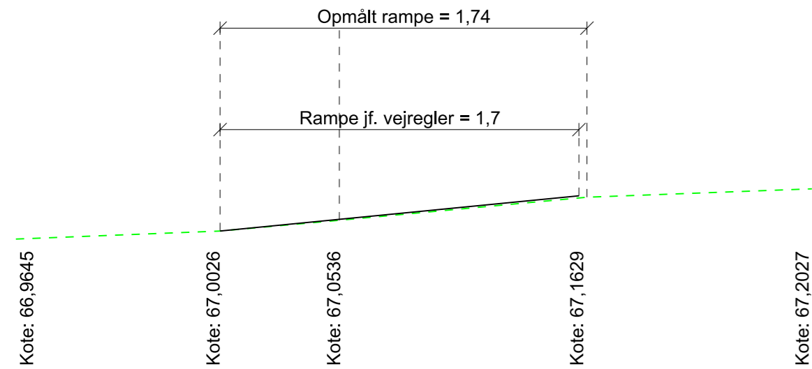
Snit M-M, 1:25 Snit igennem hævet flade nr. 05 Sydvestlig vejgren
