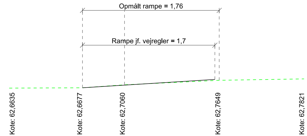
Snit A-A, 1:25 Snit igennem hævet flade nr. 01 Vestlig vejgren
