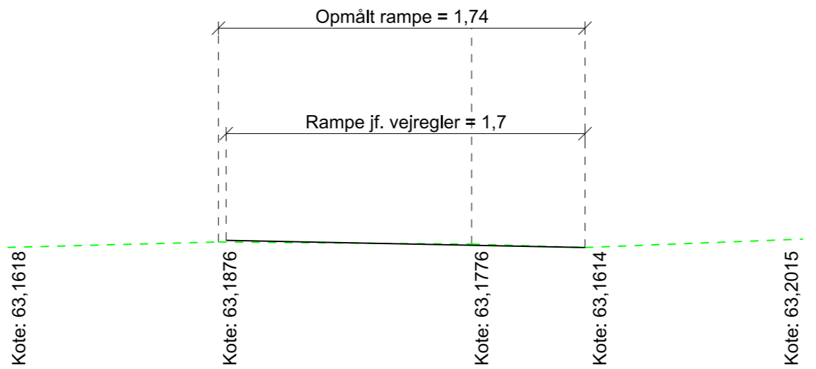
Snit B-B, 1:25 Snit igennem hævet flade nr. 01 Nordlig vejgren
