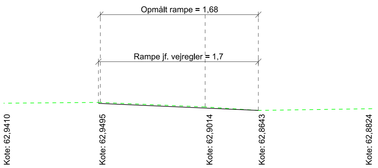
Snit C-C, 1:25 Snit igennem hævet flade nr. 01 Østlig vejgren
