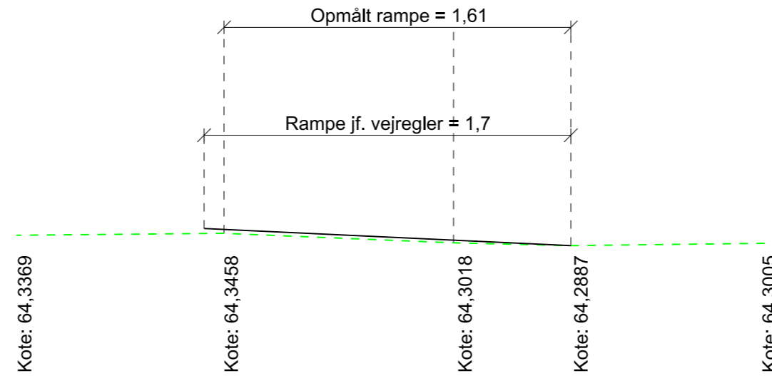
Snit E-E, 1:25 Snit igennem hævet flade nr. 02 Nordvestlig vejgren
