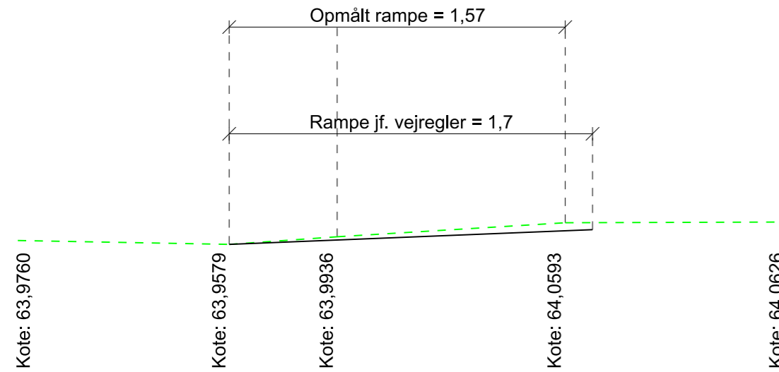
Snit D-D, 1:25 Snit igennem hævet flade nr. 02 Sydvestlig vejgren
