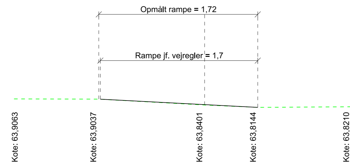
Snit I-I, 1:25 Snit igennem hævet flade nr. 03 Nordøstlig vejgren
