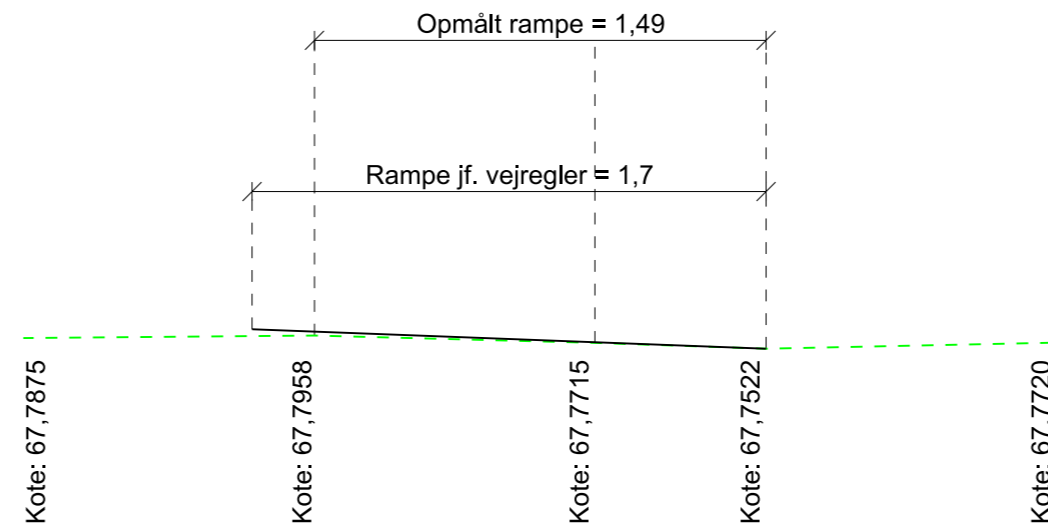
Snit N-N, 1:25 Snit igennem hævet flade nr. 05 Nordvestlig vejgren
