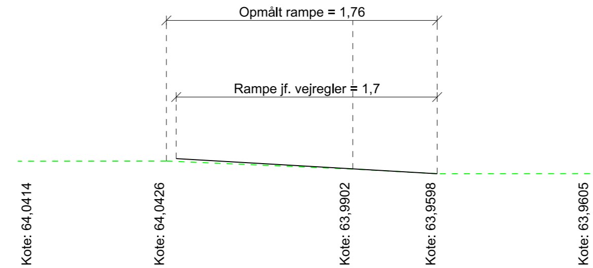
Snit H-H, 1:25 Snit igennem hævet flade nr. 03 Nordvestlig vejgren
