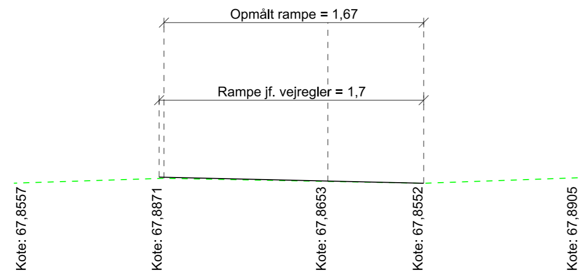
Snit O-O, 1:25 Snit igennem hævet flade nr. 05 Nordøstlig vejgren
