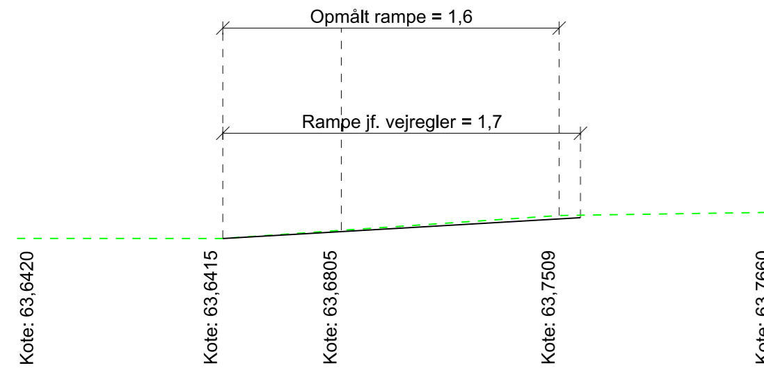
Snit G-G, 1:25 Snit igennem hævet flade nr. 03 Sydvestlig vejgren
