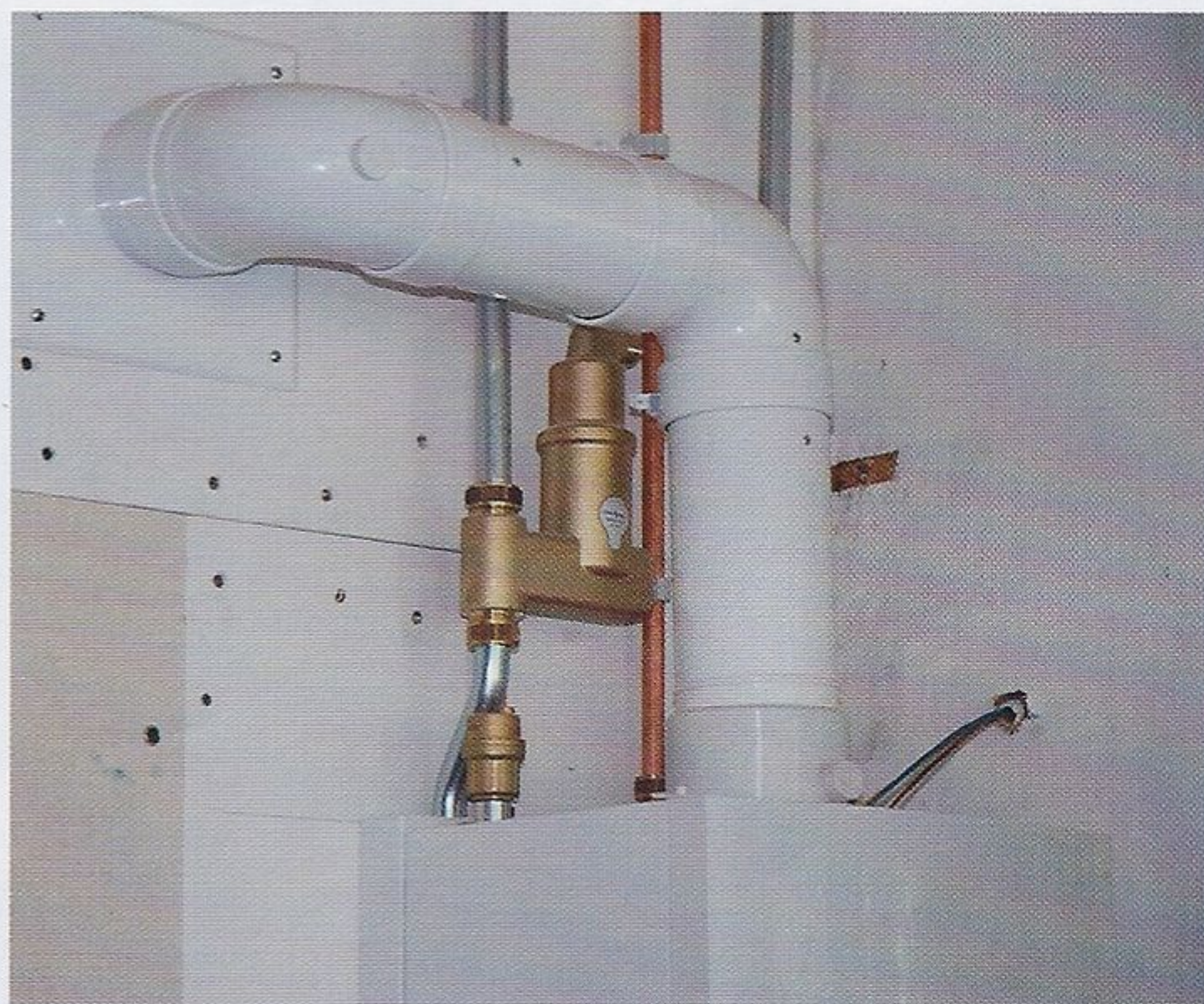
De concentrische aansluiting in de woning is de veiligste oplossing, omdat verbrandingsgassen nooit in de woning terecht kunnen komen.
