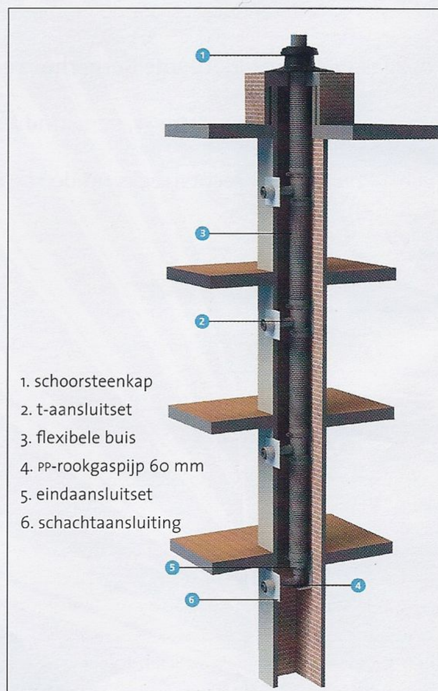
Het principe van de MultiFlex gemeenschappelijke rookgasafvoer.
