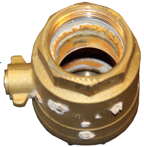
Handtaget på en förkalkad ventil har brustit och ventilihuset är korroderat på grund av avzinkning.
