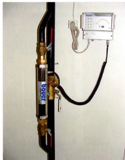
Installation med förbikoppling
