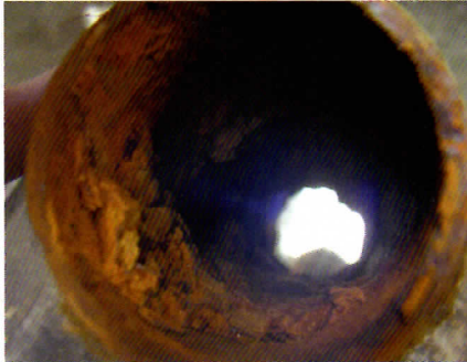
Galvaniserade kallvattenrör innan Bauer vattenbehandling har installerats
