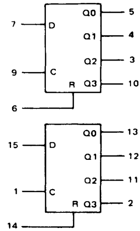
V_{DD} = Pin 16 V_{SS} = Pin 8
