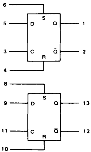
V_{DD} = Pin 14 V_{SS} = Pin 7
