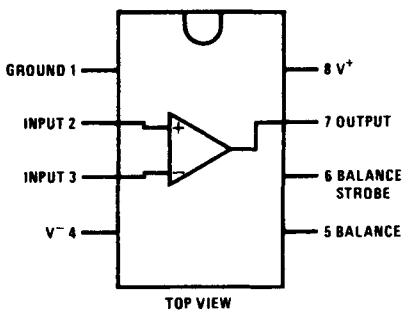
U901 MLM311
