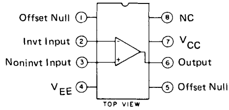
U401 MC1741CP
