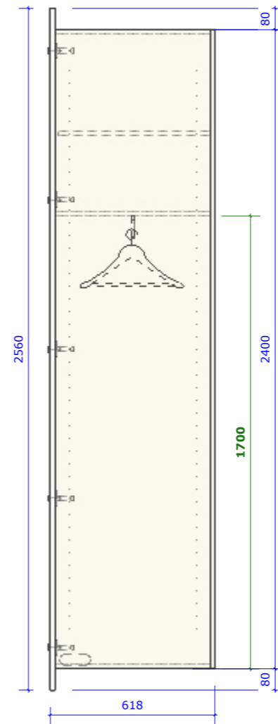
Zijaanzicht
