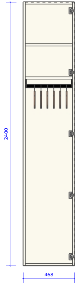
Vooraanzicht - open
