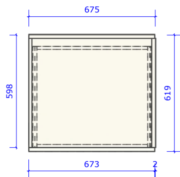
Bovenaanzicht
