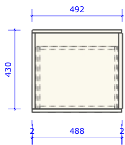
Bovenaanzicht
