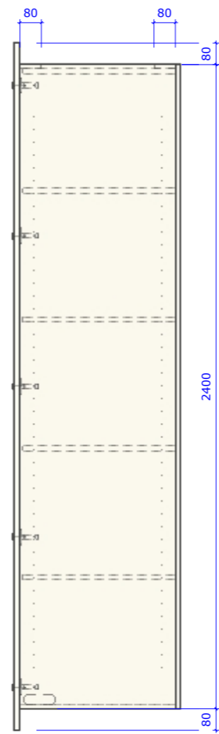
Zijaanzicht
