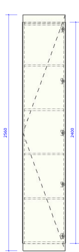
Vooraanzicht
