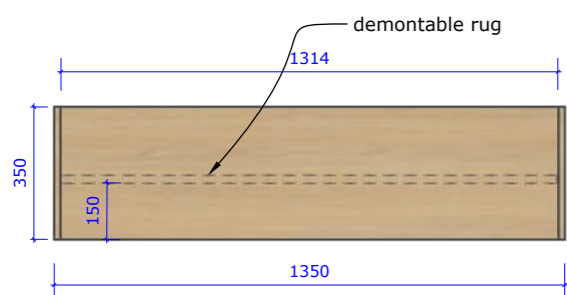
Bovenaanzicht
