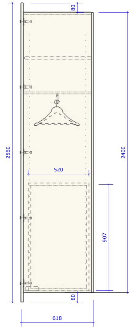
Zijaanzicht
