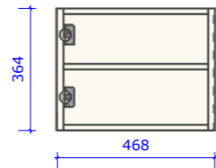
Vooraanzicht - open
