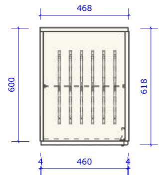
Bovenaanzicht
