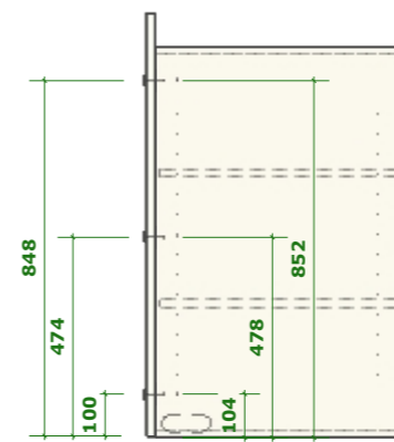
Zijaanzicht - beslagboring
