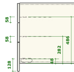
Zijaanzicht - beslagboring
