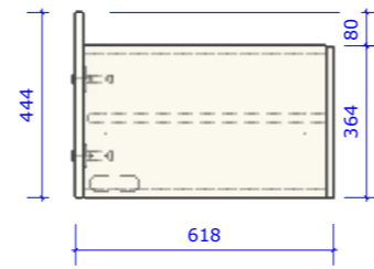
Zijaanzicht
