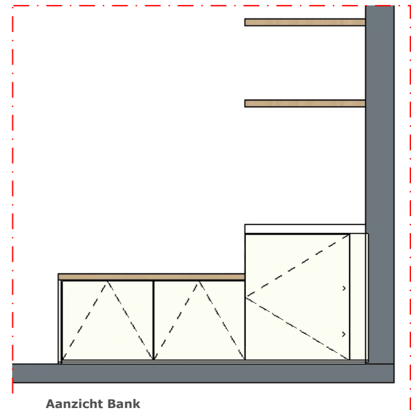
Aanzicht Bank
