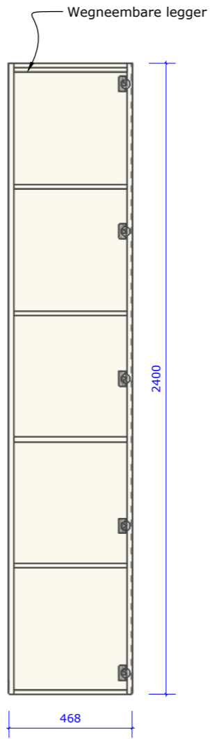
Vooraanzicht - open
