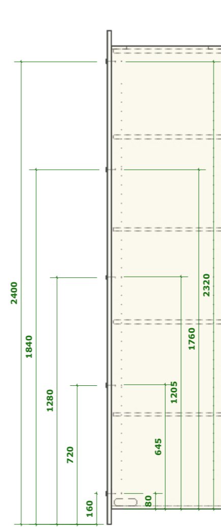
Zijaanzicht - beslagboring
