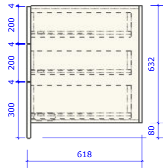
Zijaanzicht
