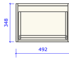
Vooranzicht - open
