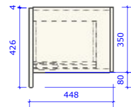
Zijaanzicht
