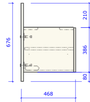
Zijaanzicht
