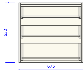
Vooraanzicht - open
