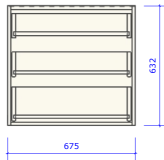
Vooraanzicht - open
