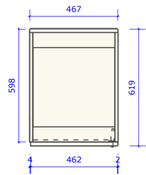
Bovenaanzicht
