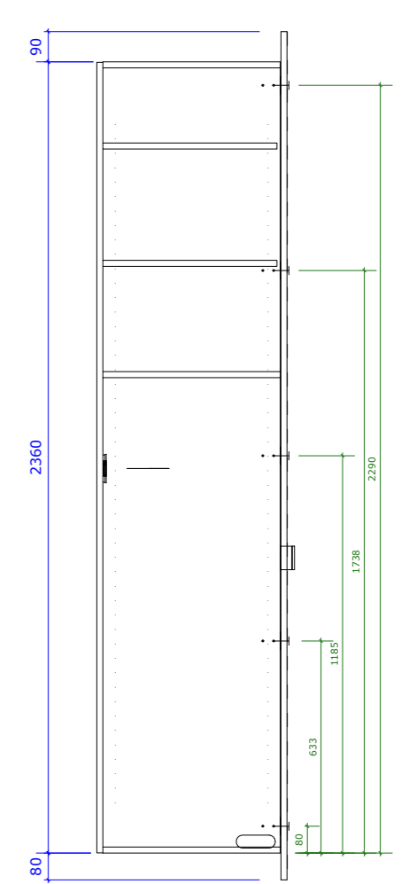
Snede
