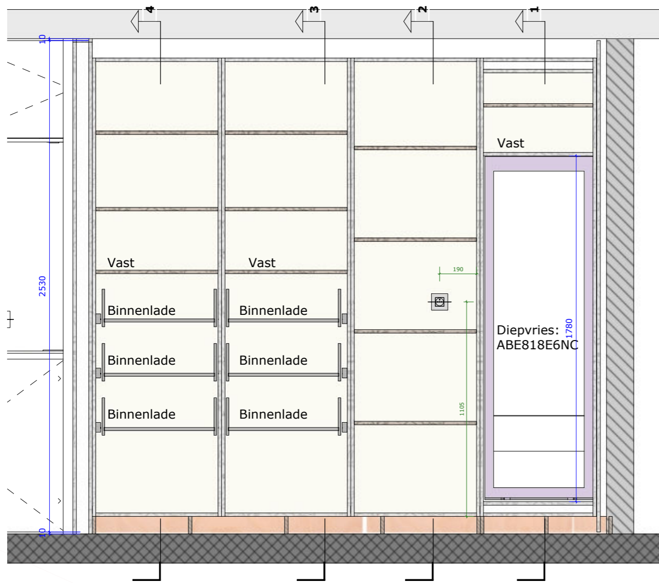
Vooranzicht
