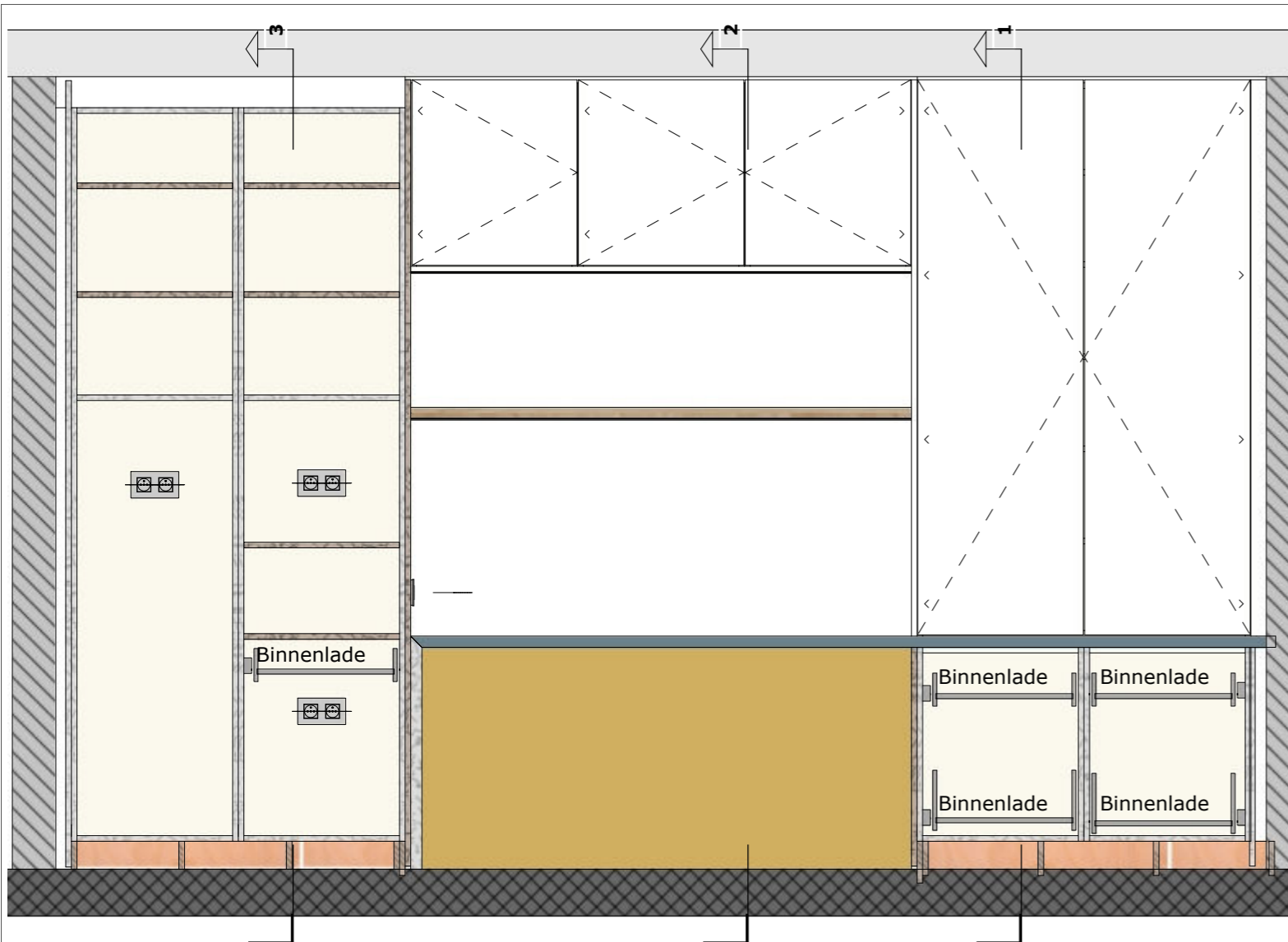
Vooranzicht
