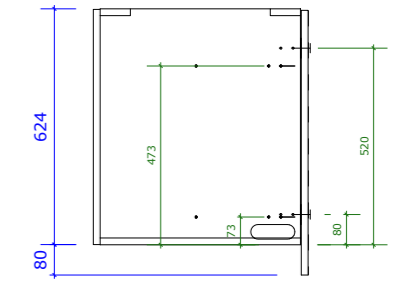
Snede
