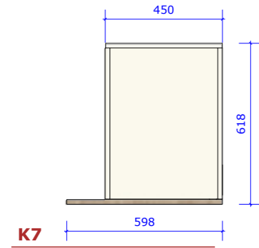
Vooraanzicht
