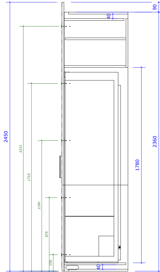
Snede
