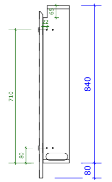
Snede
