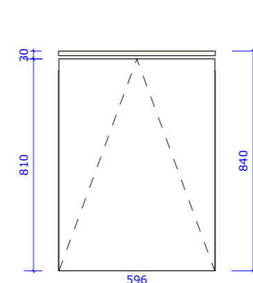
Vooraanzicht
