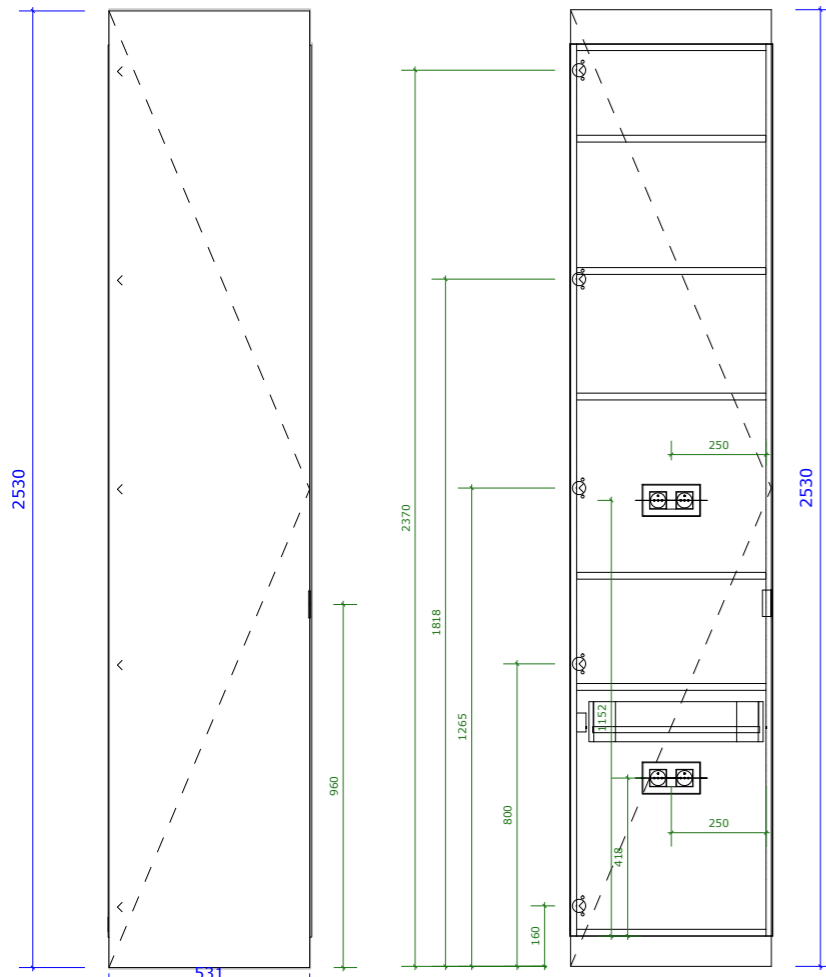
Vooranzicht
