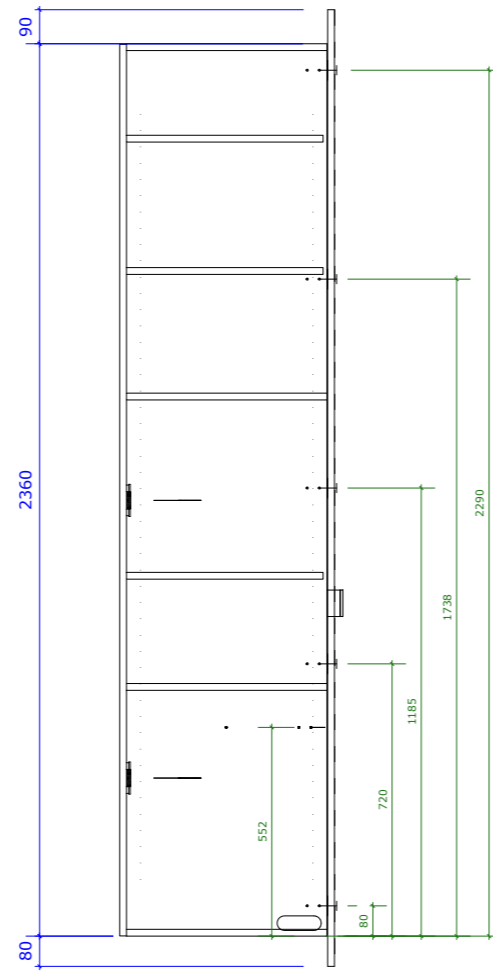
Snede
