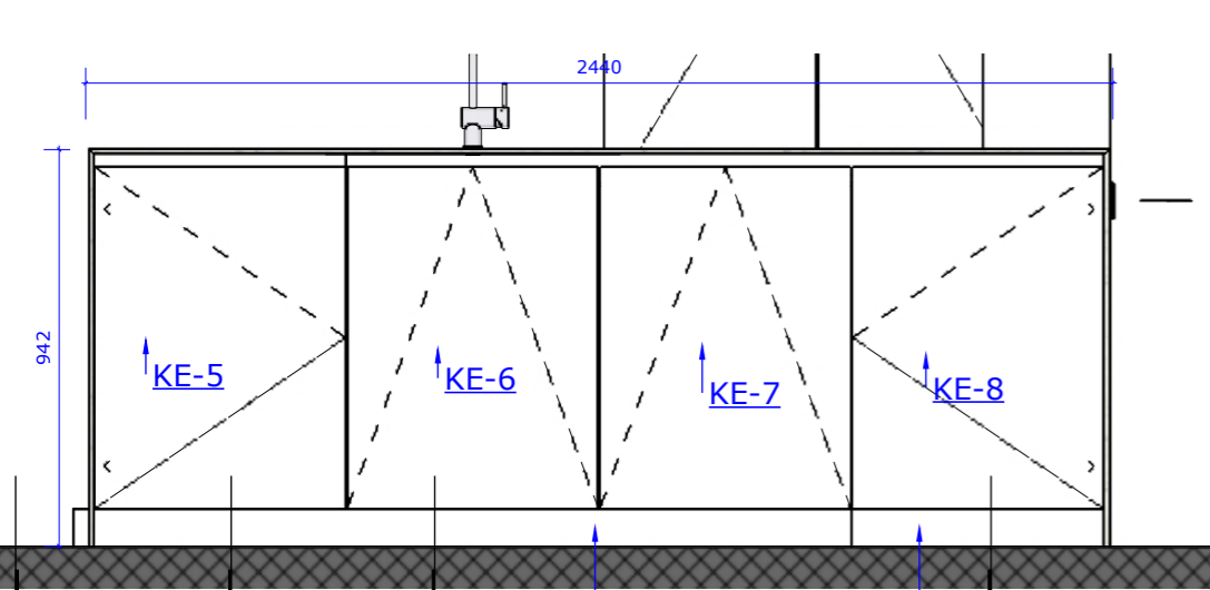
Voor aanzicht
