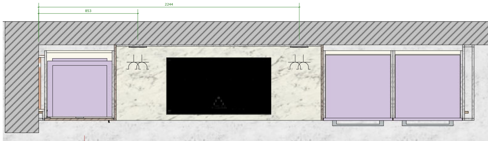
Voorzicht - indeling
