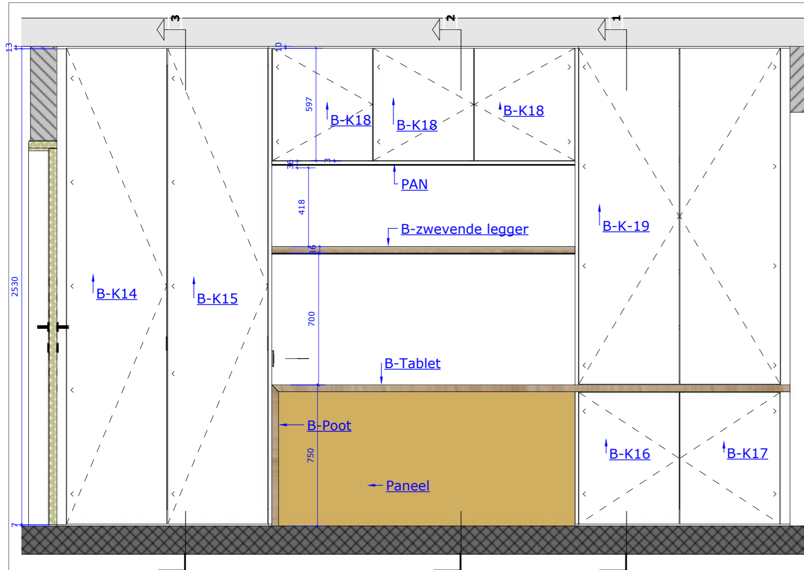
Vooranzicht
