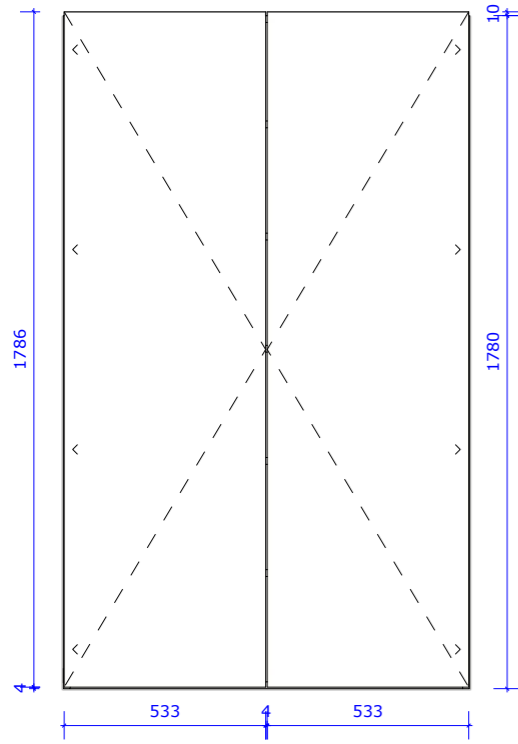
Vooraanzicht
