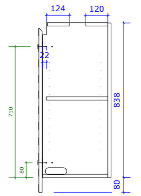
Snede
