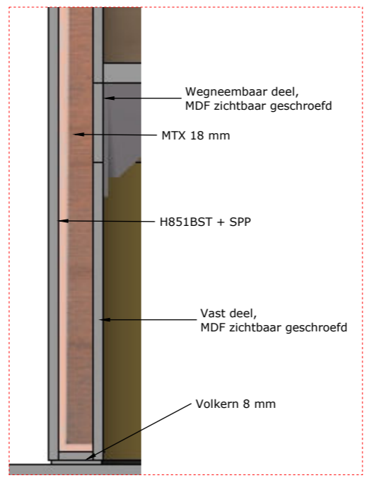
Detail rechte wandopbouw 1/10
