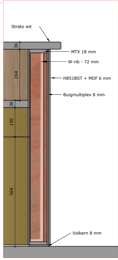
Detail gebogen wandopbouw 1/10
