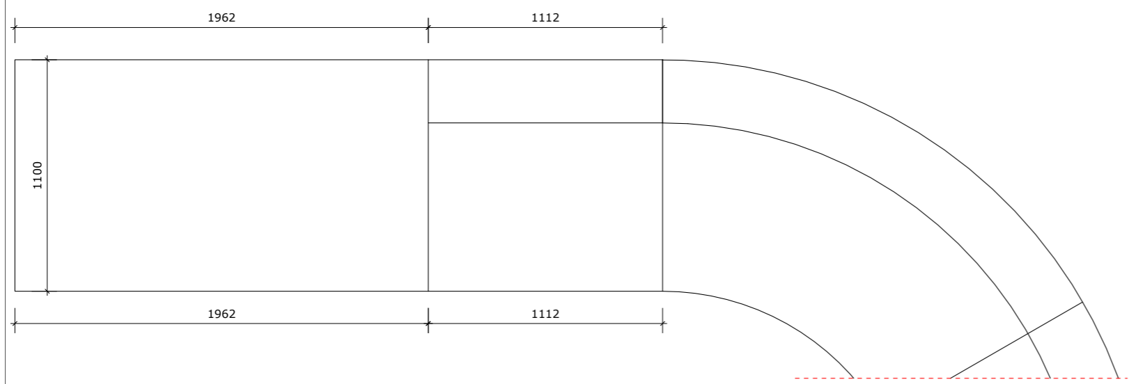
Bovenaanzicht
