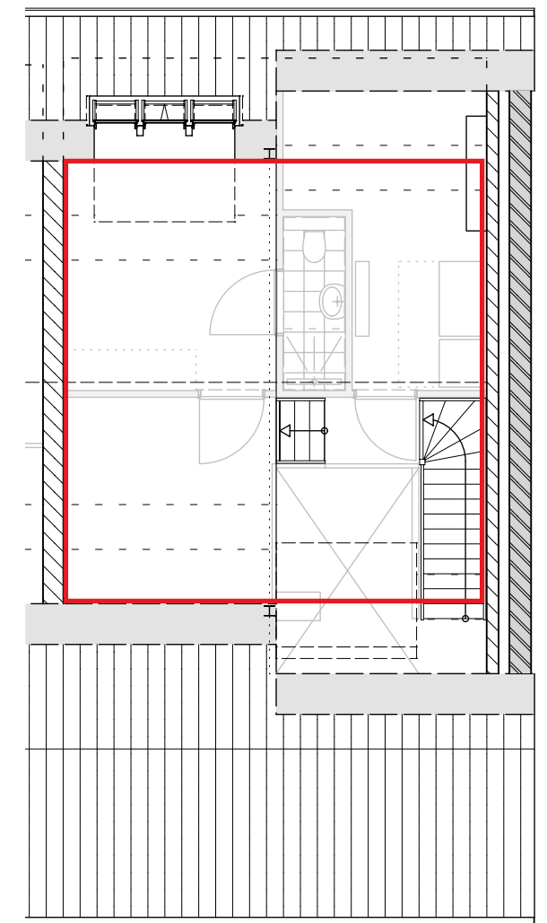
eerste verdieping
