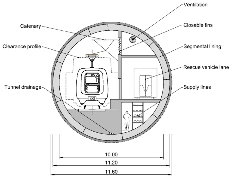
Figur 4.23 :Tværsnit af enkeltsporet tunnel med bred flugtvej.
