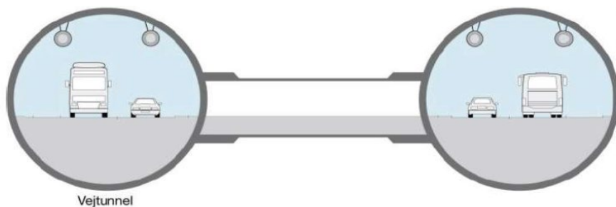
Figur 4.9: Tværsnit for den borede vejttunnel
