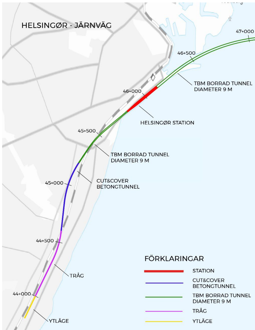
Figur 4.22: Skiss på Helsingørs station och anslutande tunnel i planläge.
