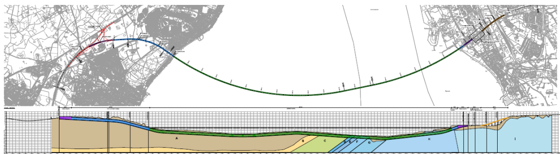
Figur 4.10: Vejforbindelsen med sænketunnel.
