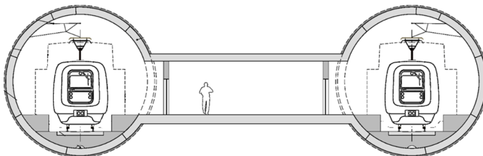
Figur 4.15: Illustrerad princip för en borrarad tunnel med två rör och tvärtunnlar.
