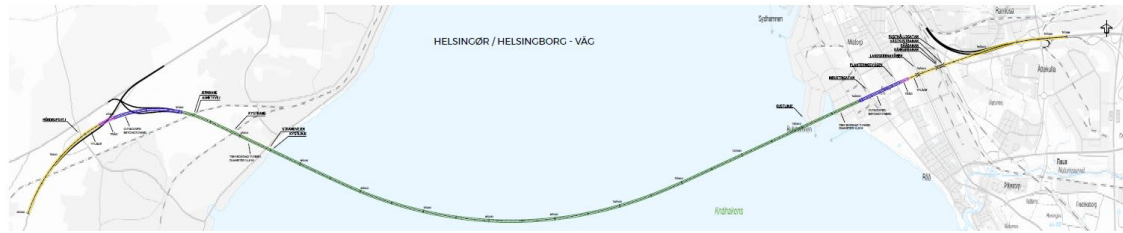
Figur 4.6: Linjeføring for vejforbindelsen i en fast HH-forbindelse.
