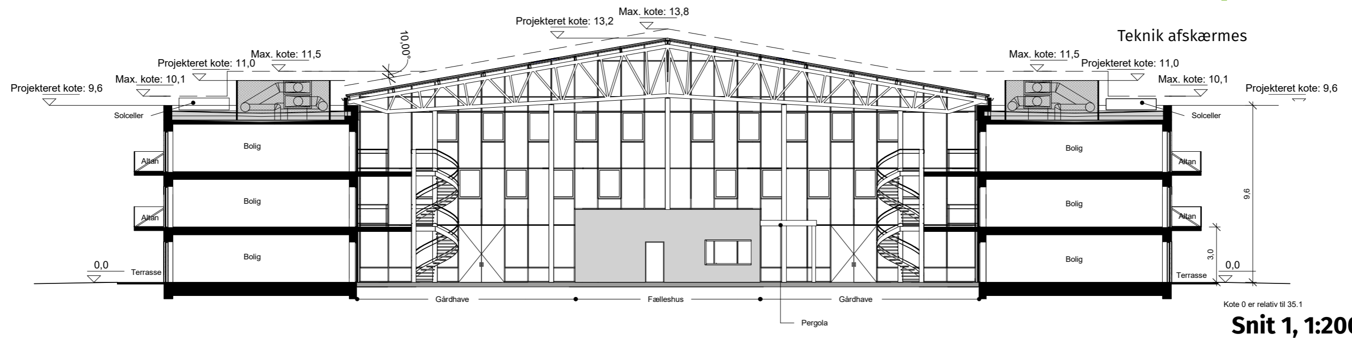
Facadesnit mod nord
