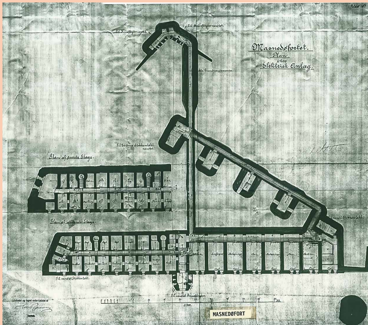
Masnedøfort er det eneste synlige danske eksempel på et trekantet stormfrit enhedsfort. Tegning fra ca. 1912, venligst udlånt af Vordingborg Lokahistoriske Arkiv.
