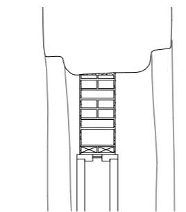
Detalj ur SD203 Skala 1:10
