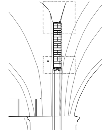
Sektionsdetalj SD202 Vägg V201, läktarplan Skala 1:20
