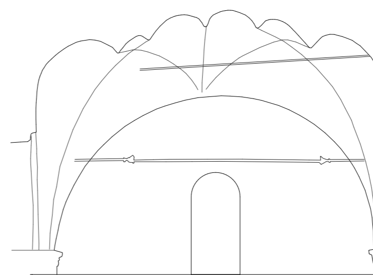
Elevationsdetalj ED202 Vägg V202, läktarplan Skala 1:20
