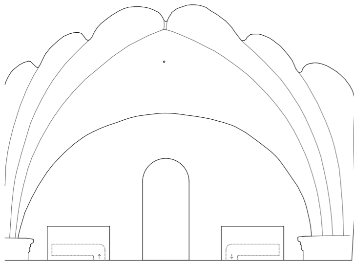
Elevationsdetalj ED201 Vägg V201, läktarplan Skala 1:20
