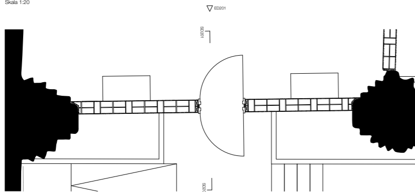
Planfigur för vägg V201, läktarplan Skala 1:20
