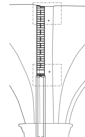
Sektionsdetalj SD204 Vägg V201, läktarplan Skala 1:20
