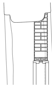
Detalj ur SD201 ovan Skala 1:10
