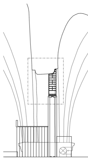
Sektionsdetalj SD201 Vägg V201, läktarplan Skala 1:20
