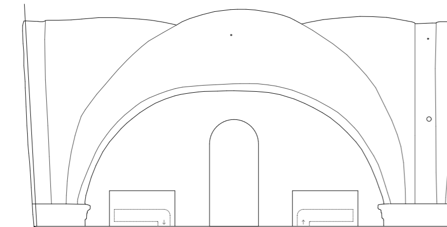
Elevationsdetalj ED203 Vägg V201, läktarplan Skala 1:20
