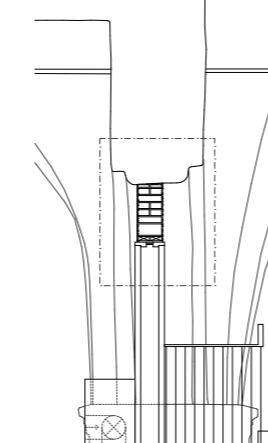
Sektionsdetalj SD203 Vägg V201, läktarplan Skala 1:20
