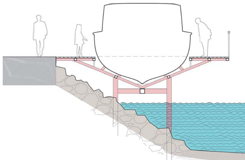
DYKARBÅTEN UNN. FÖRSLAG PÅ PLACERING INVID KAJEN FRAMFÖR DYKTANKHUSET SEKTION SKALA 1:50. BSK ARKITEKTER / SBN 09-03-25
