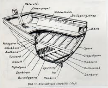
Bild 31. Kravellbyggd skeppsbåt (slup)
