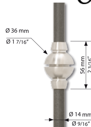
AISI 304 (V2A) WM 54 AISI 316 (V4A) WM 954
