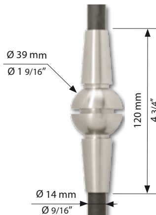
AISI 304 (V2A) WM 124 AISI 316 (V4A) WM 9124
