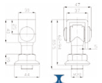
SH 155-20 150 Kg 330 lb
