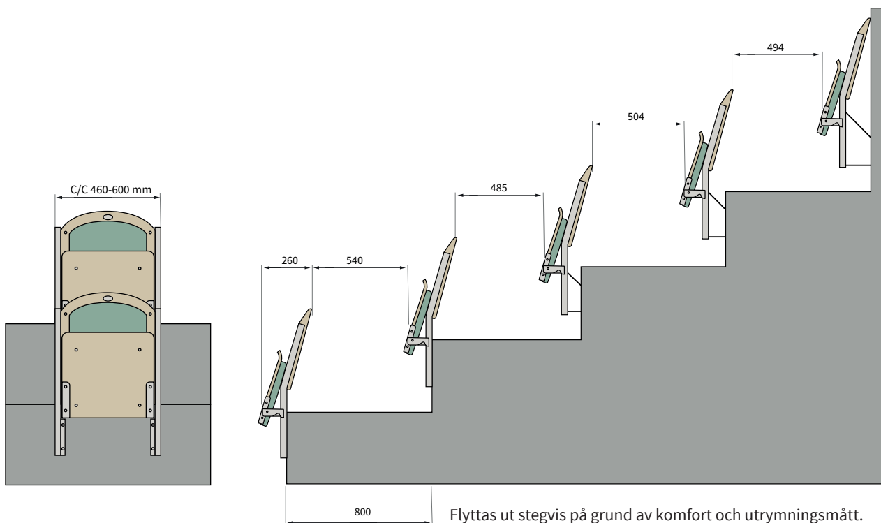
Stadion Comfort med dubbla fjädrar. Måttskissen är för 450 millimeter hög gradäng.
