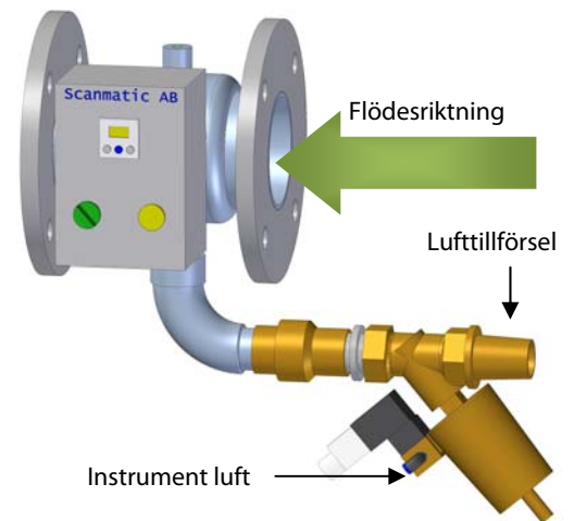
Ringejektor med luftarrangemang och styrning
