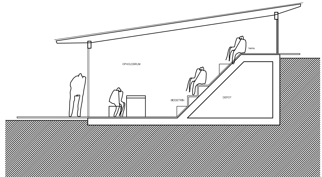
Snit 1:100
