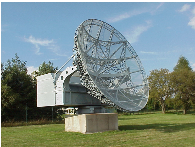
Würzburg-Riese.
