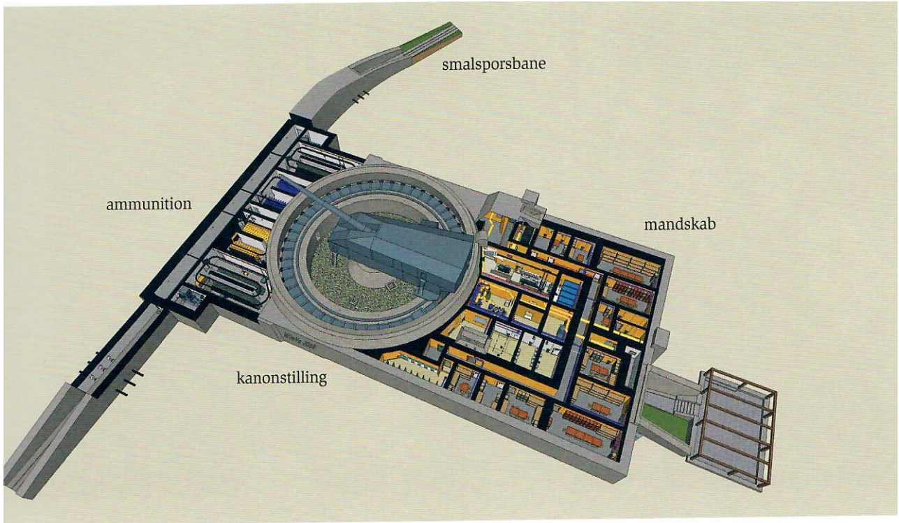
38 cm kanonstilling
