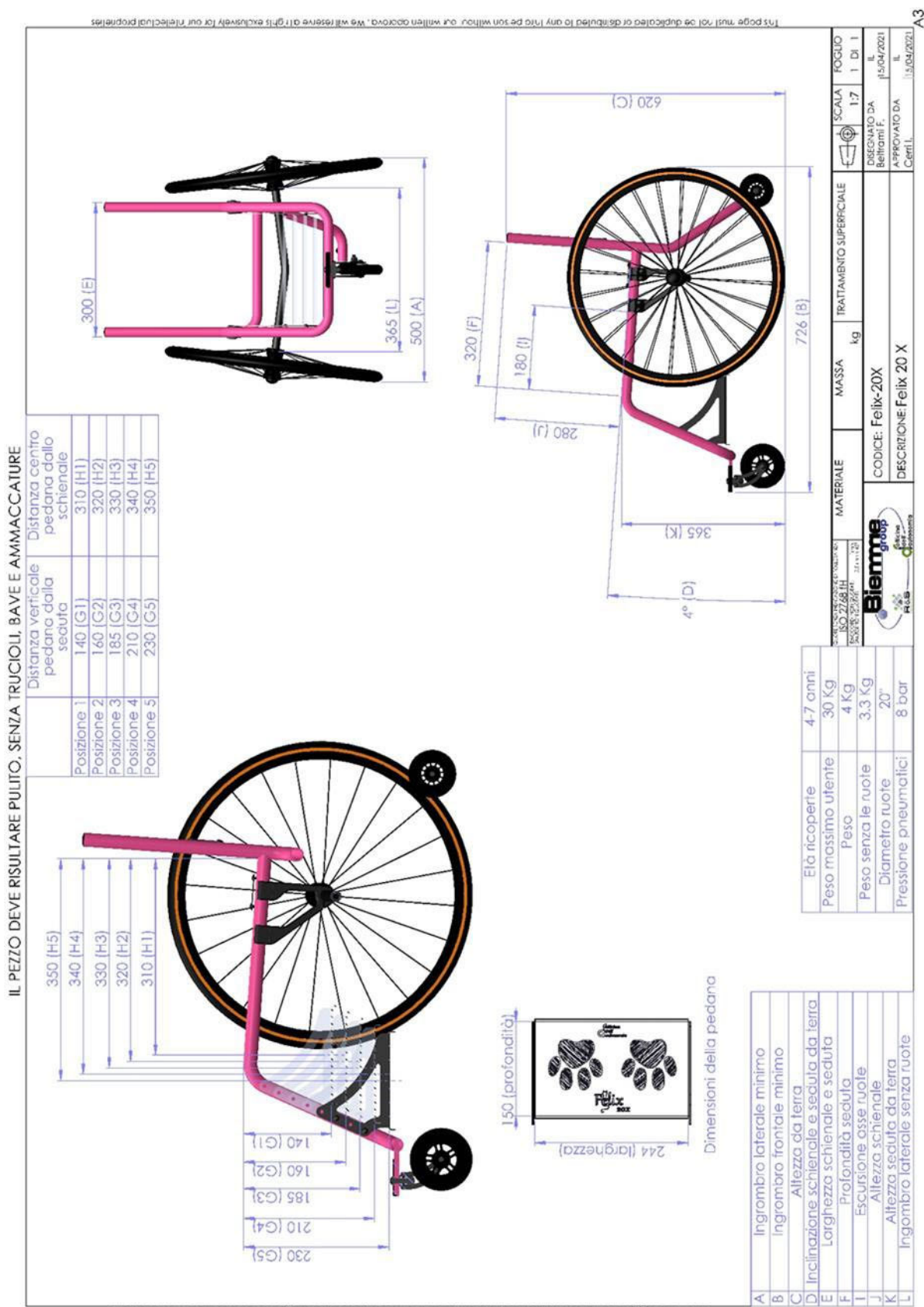
Fig. 3 – Desenho técnico FELIX 20X
