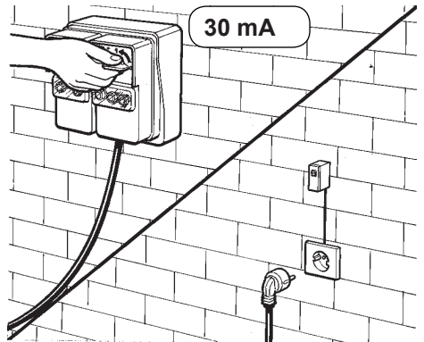
Sähkökytkentä.
