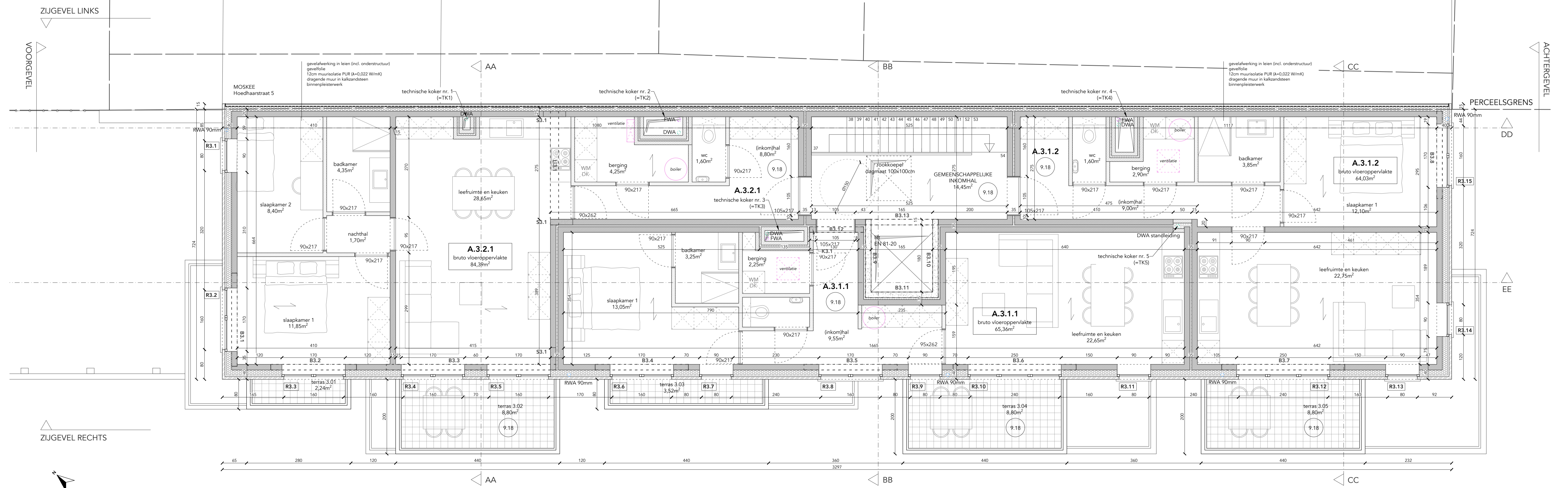
PLAN VERDIEPING +3 nieuwe toestand schaal 1/50
