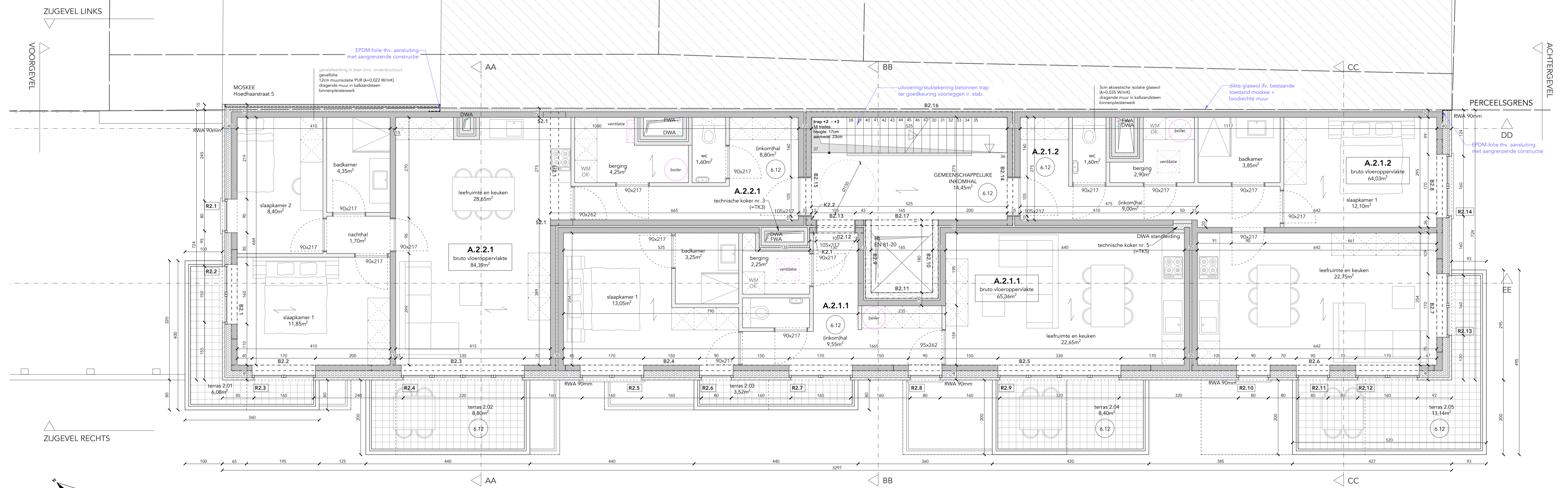
PLAN VERDIEPING +2 nieuwe toestand schaal 1/50
