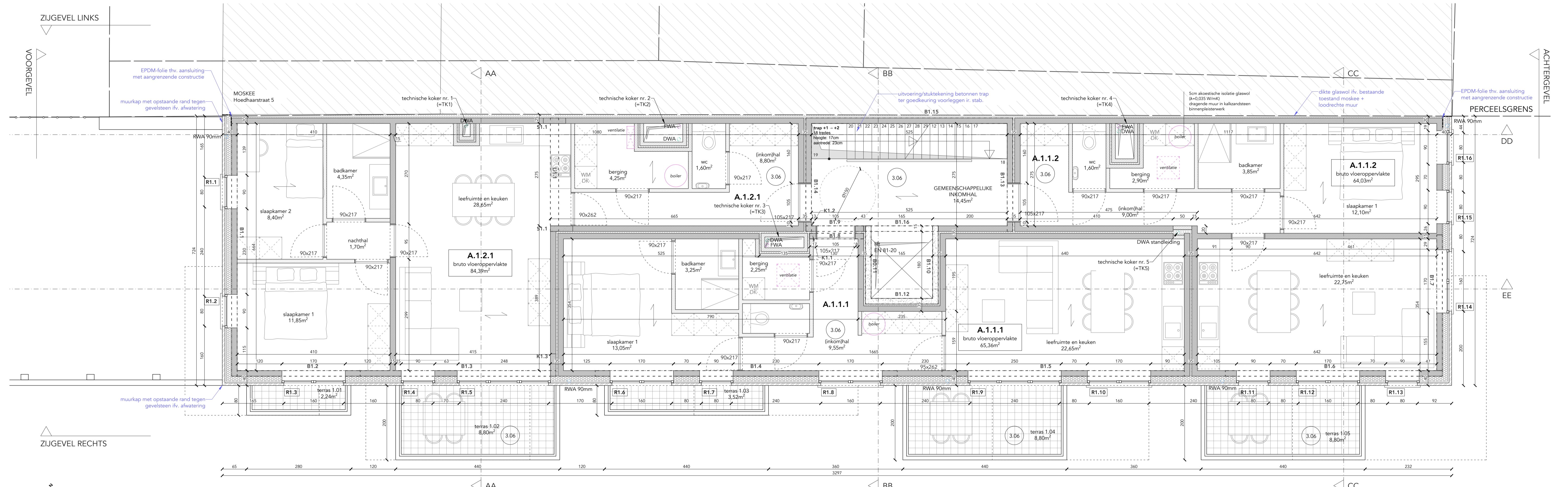
PLAN VERDIEPING +1 nieuwe toestand schaal 1/50
