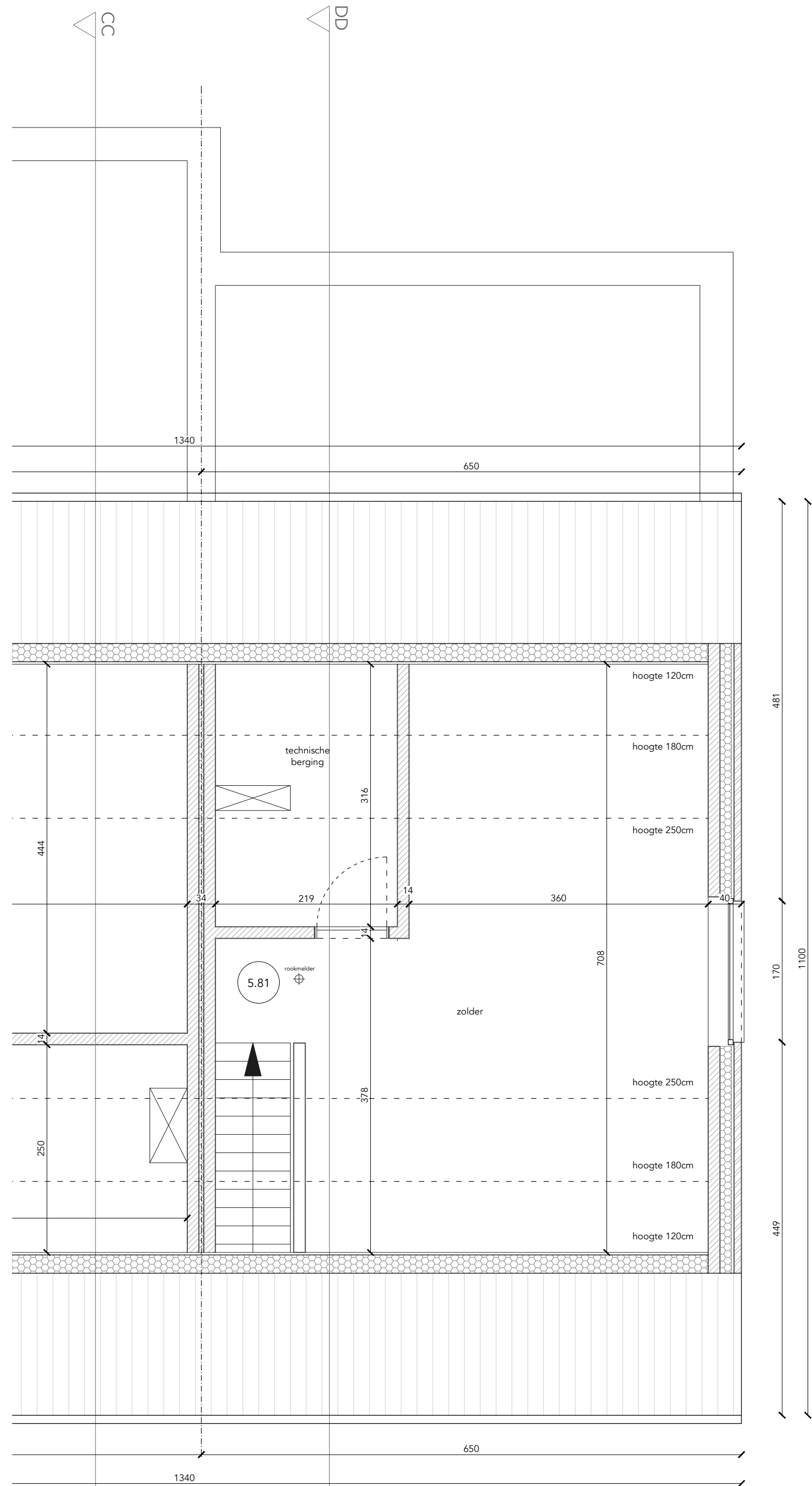
ZOLDERPLAN (schaal 1/50)
