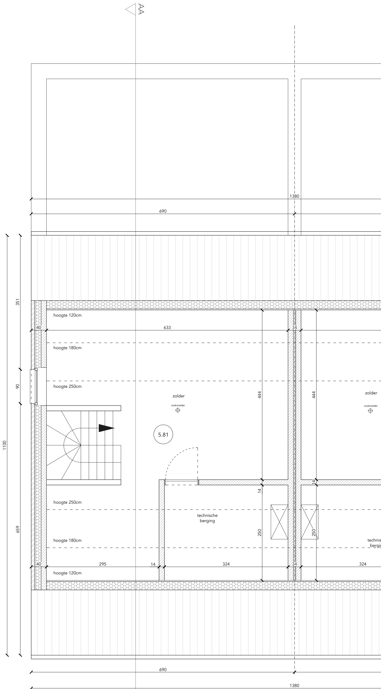
ZOLDERPLAN (schaal 1/50)
