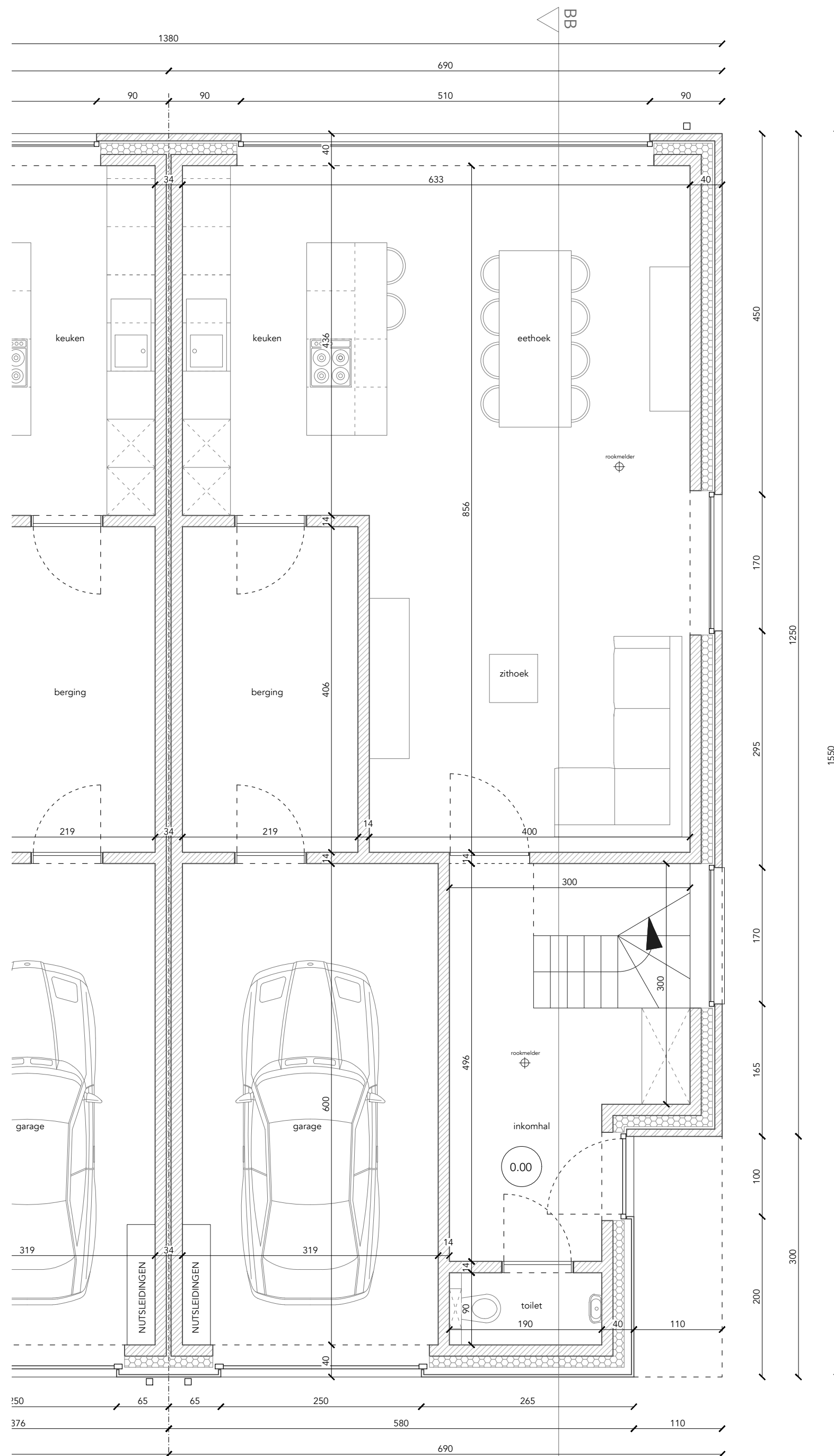
PLAN GELIJKVLOERS (schaal 1/50)
