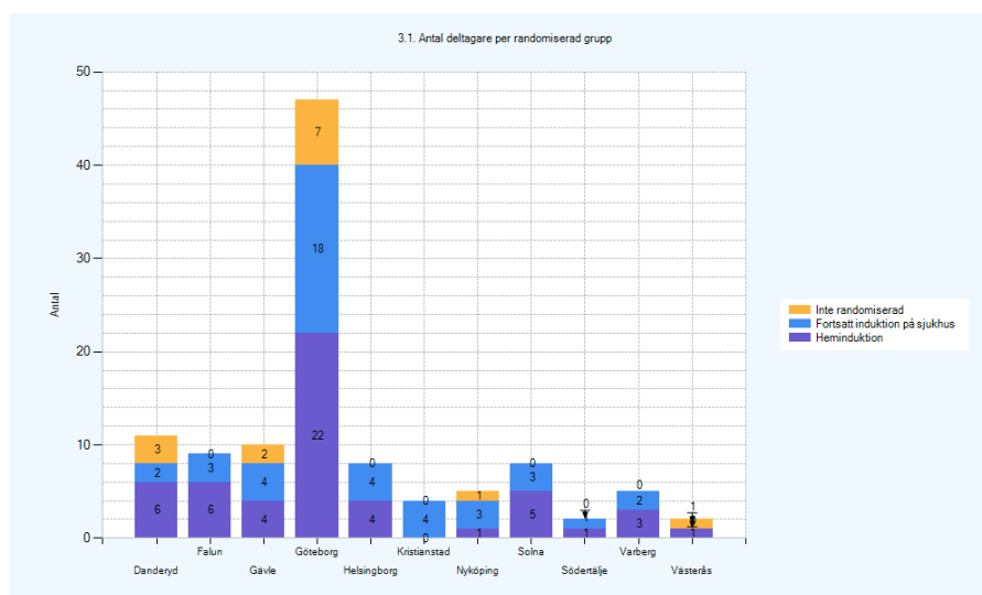
3.1. Antal deltagare per randomiserad grupp
