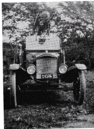
Kolind Brandvæsens første motorsprøjte fra 1925. Den er bygget over et Ford T chassis af brandinspektør og snedkermester A.C.Hansen og maskinsmed Oskar Jensen på sidstnævntes værksted i Kolind. - Stående bag sprøjten: snedkermester A.C.Hansen. På førersædet: vognmand O.Kjeldsen og blikkenslager R.M.Jensen. På mandskabssædet: murer Rs.Holst, karetmager J.P.Sørensen og maskinsmed Oskar Jensen.
