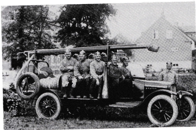
Kolind Brandvæsens første motorsprøjte fra 1925. Den er bygget over et Ford T chassis af brandinspektør og snedkermester A.C.Hansen og maskinsmed Oskar Jensen på sidstnævntes værksted i Kolind. - Stående bag sprøjten: snedkermester A.C.Hansen. På førersædet: vognmand O.Kjeldsen og blikkenslager R.M.Jensen. På mandskabssædet: murer Rs.Holst, karetmager J.P.Sørensen og maskinsmed Oskar Jensen.
