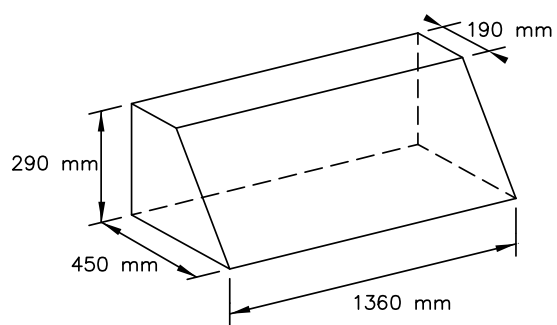
Dessin/Drawing 279-4
