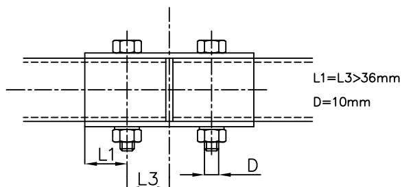
Dessin/Drawing 253-42
