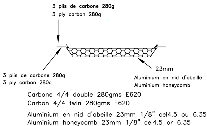
Dessin/Drawing 255-14
