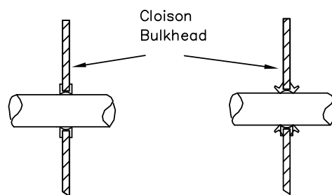
Dessin/Drawing 253-60
