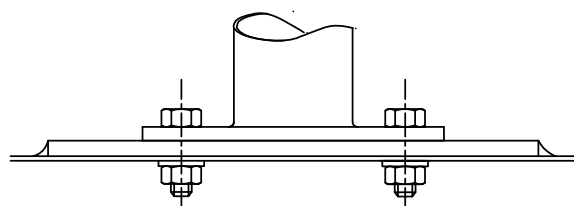
Dessin/Drawing N°253-51
