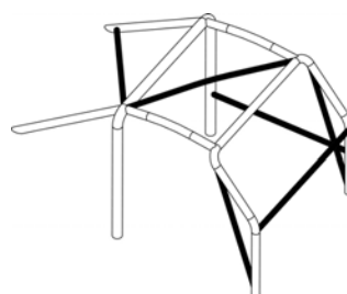
Dessin/Drawing 283-2
