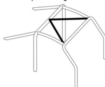
Dessin/Drawing 253-14
