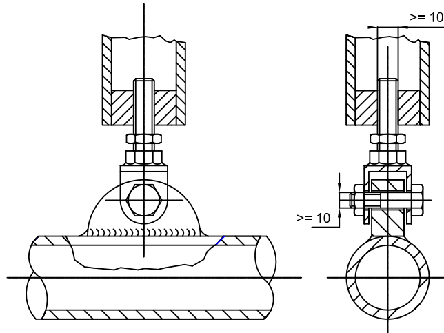
Dessin/Drawing 253-47
