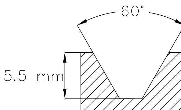
Dessin/Drawing 279-5
