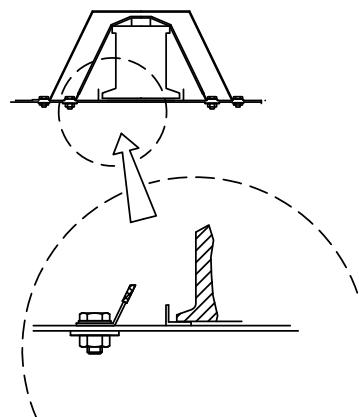
Dessin/Drawing 255-8
