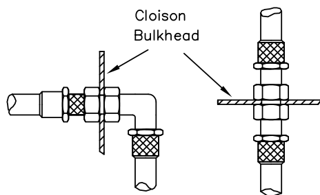
Dessin/Drawing 253-59
