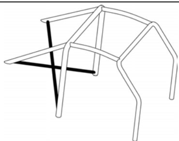
Dessin/Drawing 253-19
