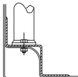
Dessin/Drawing 253-55
