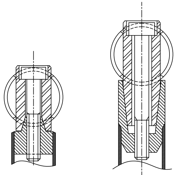
Dessin/Drawing 253-38 Dessin/Drawing 253-39
