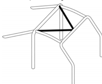
Dessin/Drawing 253-13
