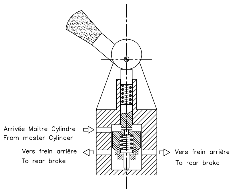
Dessin/Drawing N°263-9
