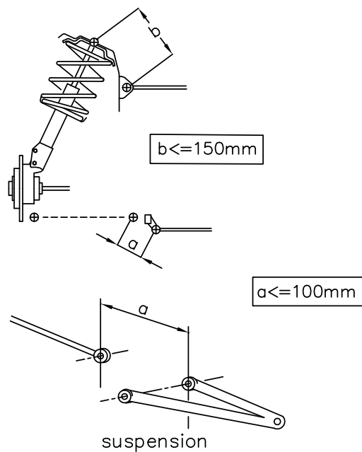
Dessin/Drawing 255-4
