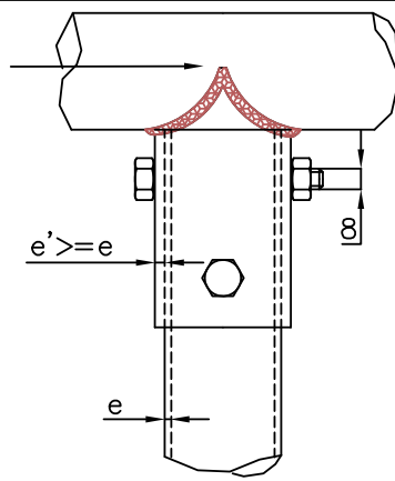
Dessin/Drawing 253-44
