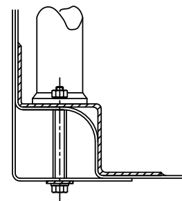
Dessin/Drawing 253-56
