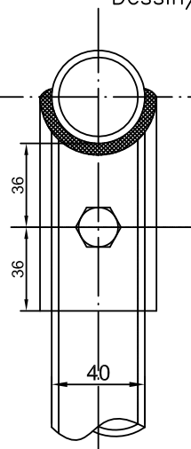
Dessin/Drawing 253-45
