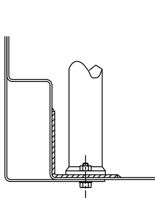
Dessin/Drawing 253-53
