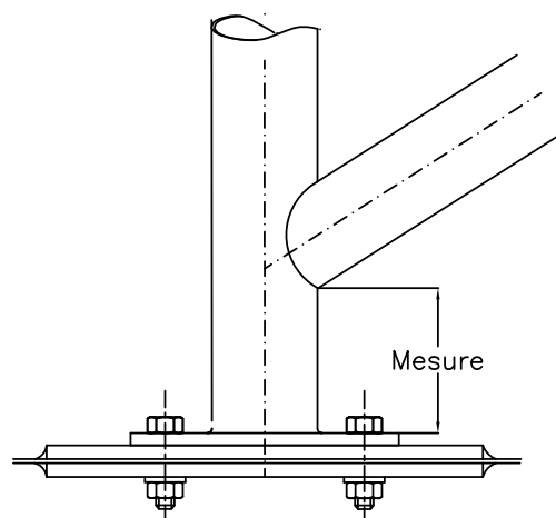
Dessin/Drawing 253-52
