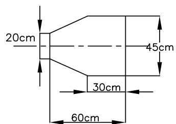
Dessin/Drawing 259-2
