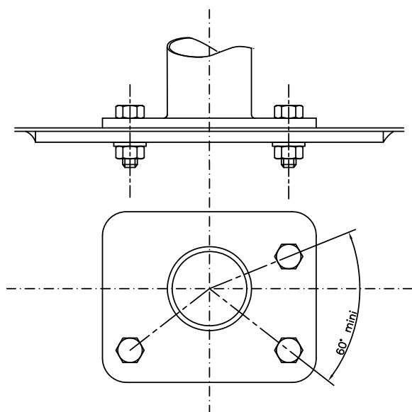
Dessin/Drawing 253-50
