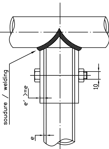
Dessin/Drawing 253-45
