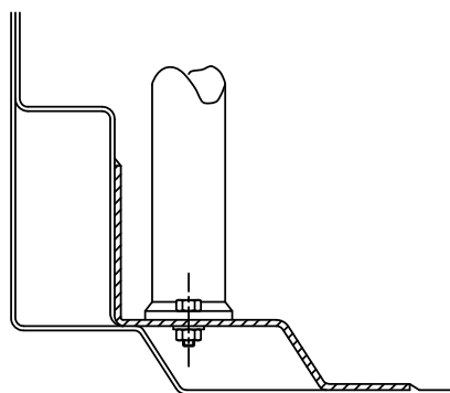
Dessin/Drawing 253-54
