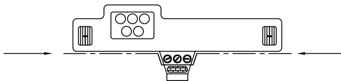
Dessin/Drawing 255-7
