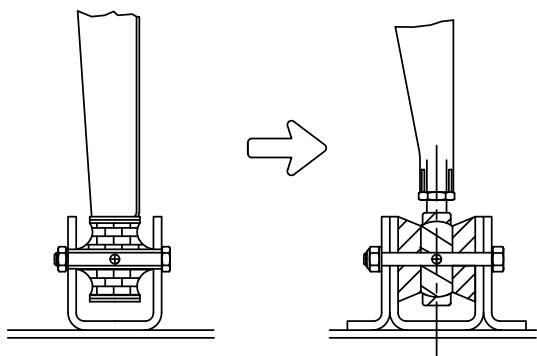
Dessin/Drawing 255-5
