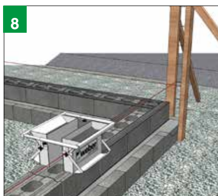
8 Lägg på Weber Flexoheft med Leca Murlåda.
