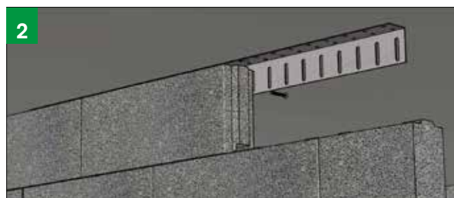
2 Lägg på Weber Flexoheft och stapla upp sista skiftet. Fäst blocken i takprofilen med Therm 406 Träskruv 4,8 x 45.
