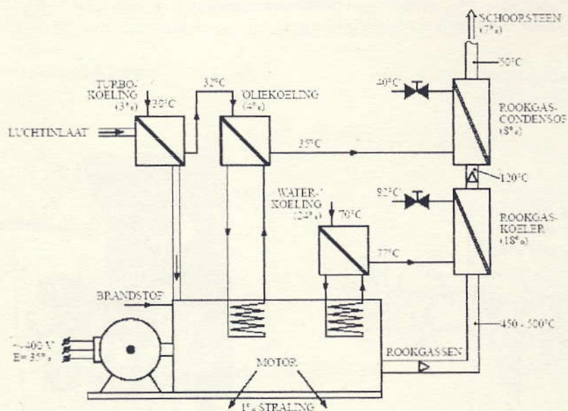
Figuur 2.1. Motortoepassing voor WKK
