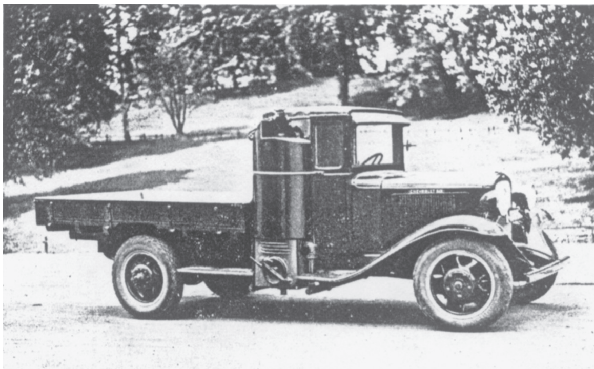
Lastebil med norskbygd trekull-gassgenerator.
