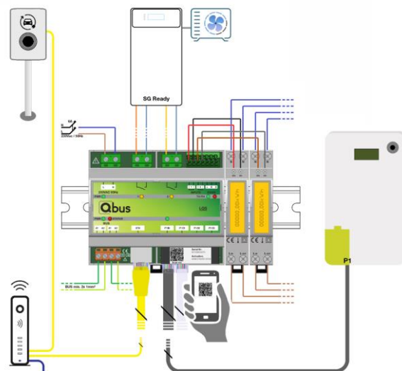
Figuur 3 Aansluitschemavoorbeeld
