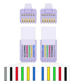
Figuur 5 Fiches gekruiste RJ12-kabel
