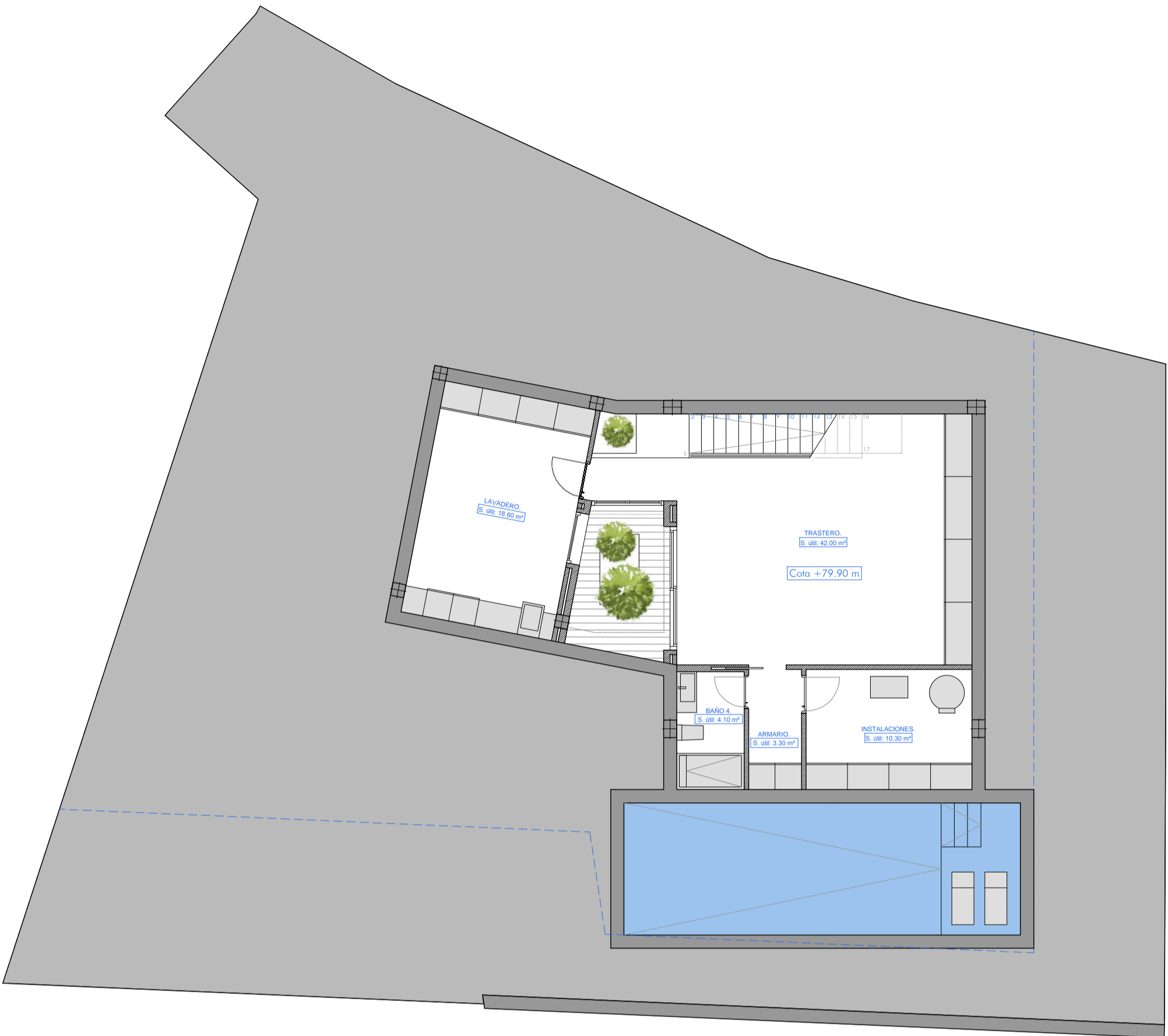
PLANTA SÓTANO: Superficie construida: 93.80 m 2
