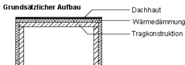
Abbildung 11 unbelüftetes Flachdach
