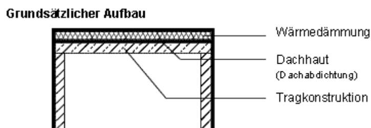
Abbildung 12: unbelüftetes Umkehrdach
