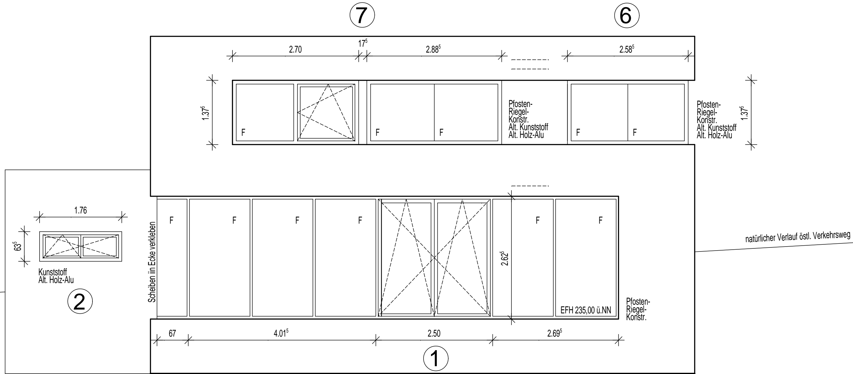
West-Ansicht
