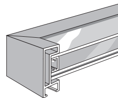
PROFIL 2253 (Profil 225 + 223 Entre-deux-verres)
