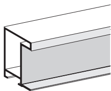
PROFIL 222 25x45 mm / F=35,5 mm
