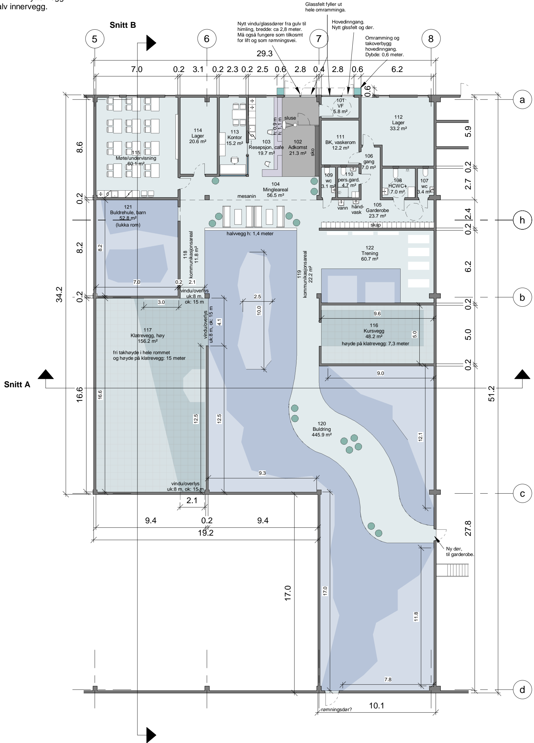
Klatrehall i Ellobygget Målsatt planskisse 29.10.20 1:200, A3
