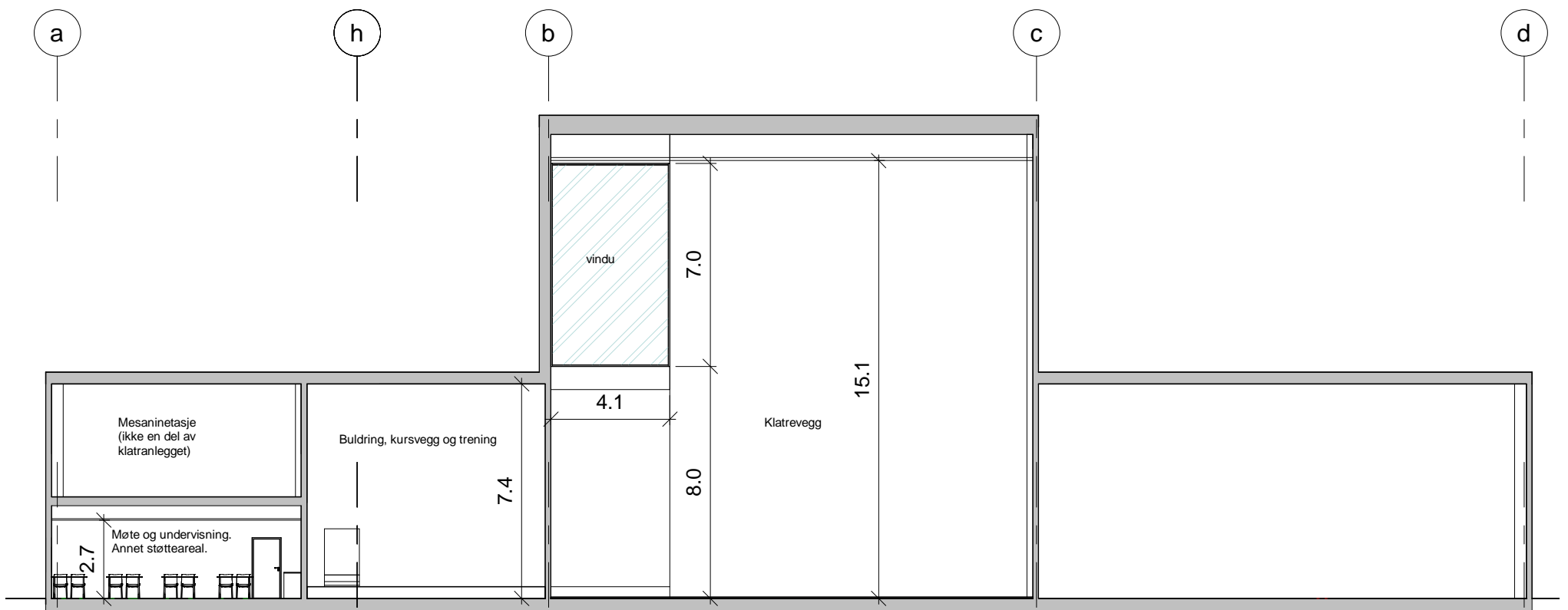
Snitt A
