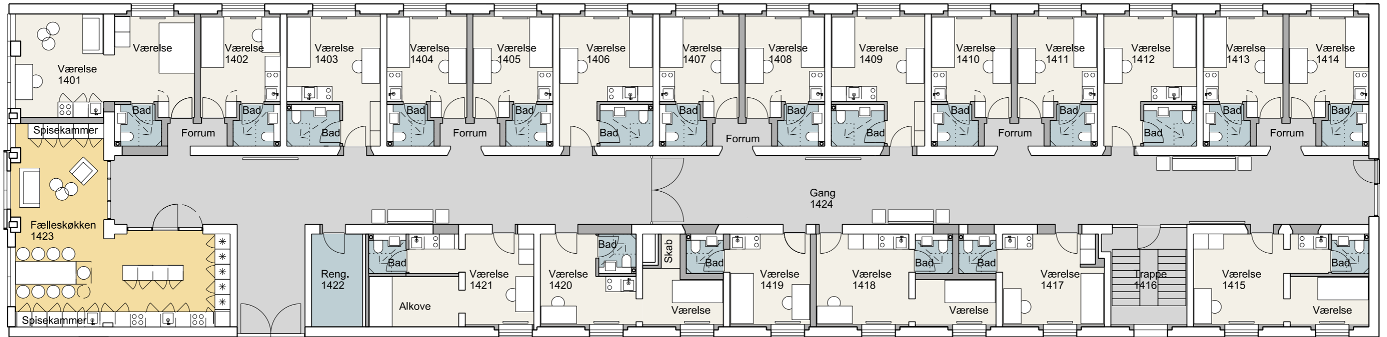
Plan, etage 4
