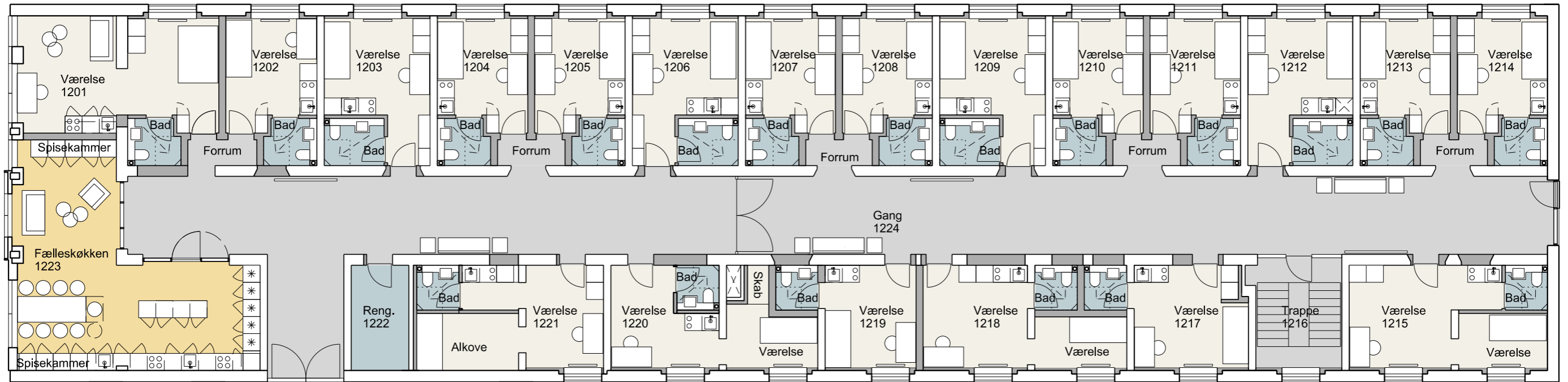
Plan, etage 2
